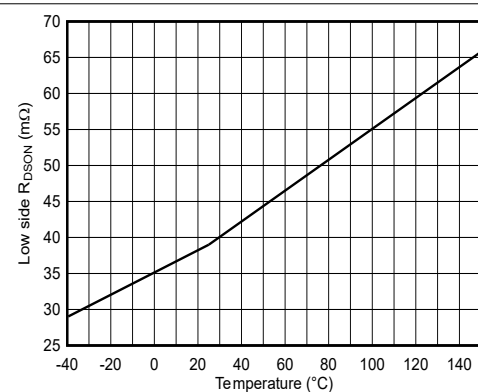
図 6-4. ローサイド MOSFET の R_{DS-ON}
