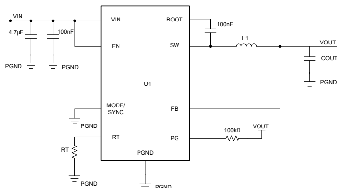
図 8-21. アプリケーション回路例
