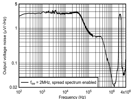
LMR61440-Q1 F SW = 2MHz 3.3V 出力 I OUT = 4A V IN = 12V
