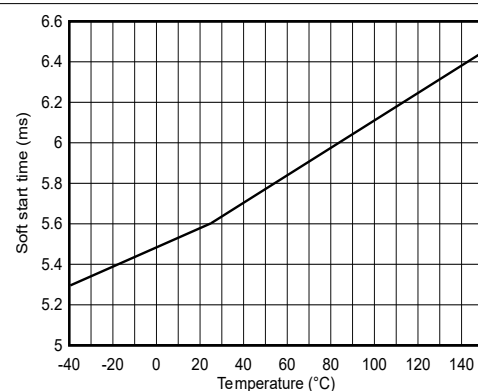
図 6-6. ソフトスタート時間
