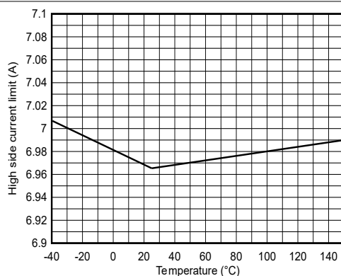
図 6-1. ハイサイド MOSFET 電流制限
