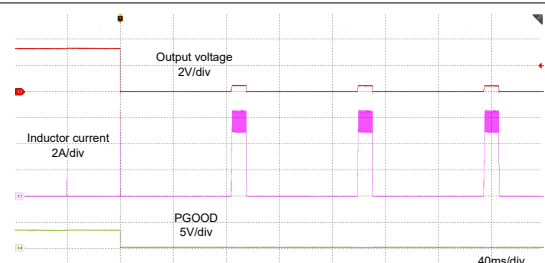
LMR61440-Q1 3.3V 固定出力 モード = 自動 F_{SW} = 2\text{MHz} V_{IN} = 24\text{V}
