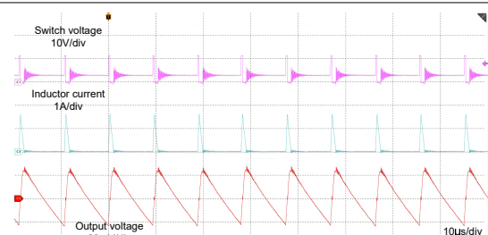
LMR61440-Q1 3.3V 出力 モード = 自動 I_{OUT} = 100\text{mA} F_{SW} = 2\text{MHz} V_{IN} = 12\text{V}
