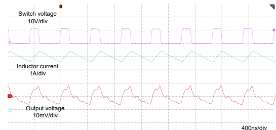
LMR61440-Q1 3.3V 出力 モード = FPWM I_{OUT} = 4\text{A} F_{SW} = 2\text{MHz} V_{IN} = 12\text{V}
