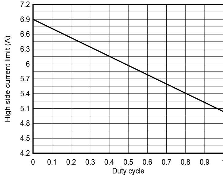
図 7-4. デューティ サイクル D の関数としての典型的なハイサイド電流制限 I_{HS-LIM}
