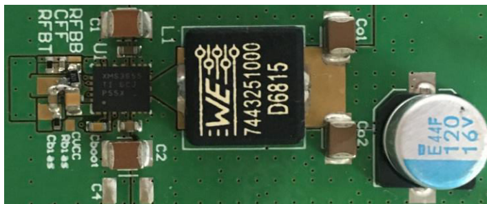
图 11-3. LMS3655MQEVM Layout
