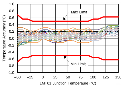
LMT01の精度
