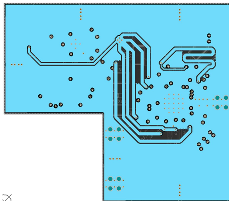
図 96. Mid Layer 1
