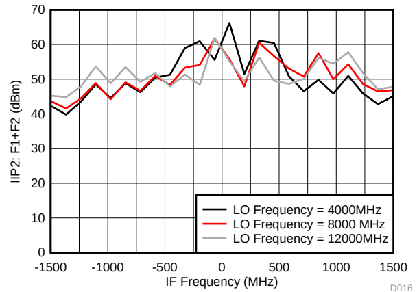
FIG 16. IIP2: F1+F2 Across LO Frequency for External LO Mode
