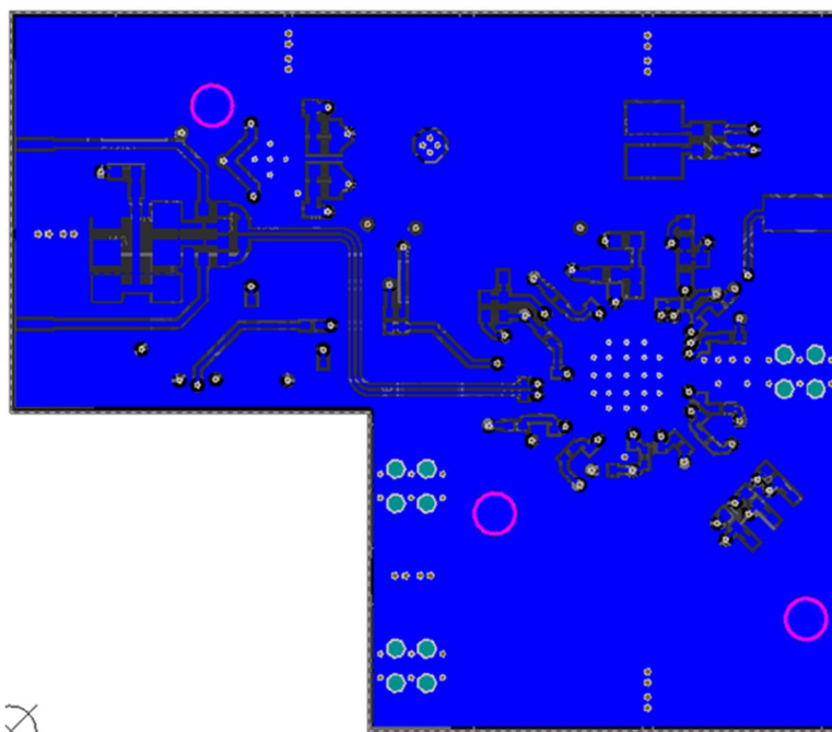
図 99. Bottom Layer
