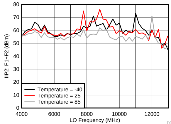
FIG 16. IIP2: F1+F2 Across LO Frequency for External LO Mode
