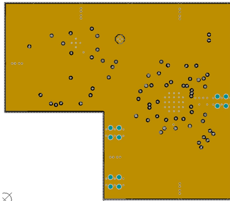
図 95. Ground Layer 1
