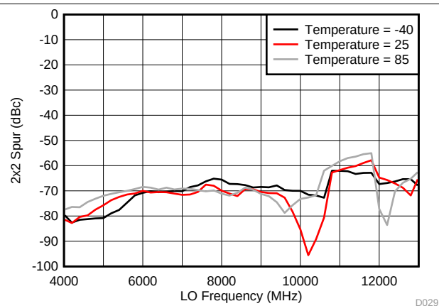
FIG 32. 2x2 Spur for Internal LO Mode
