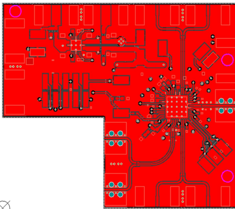
✕ 94. Top Layer
