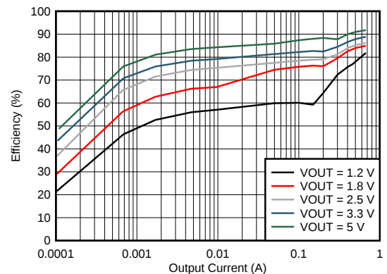
V_{IN} = 12\text{ V} での効率
