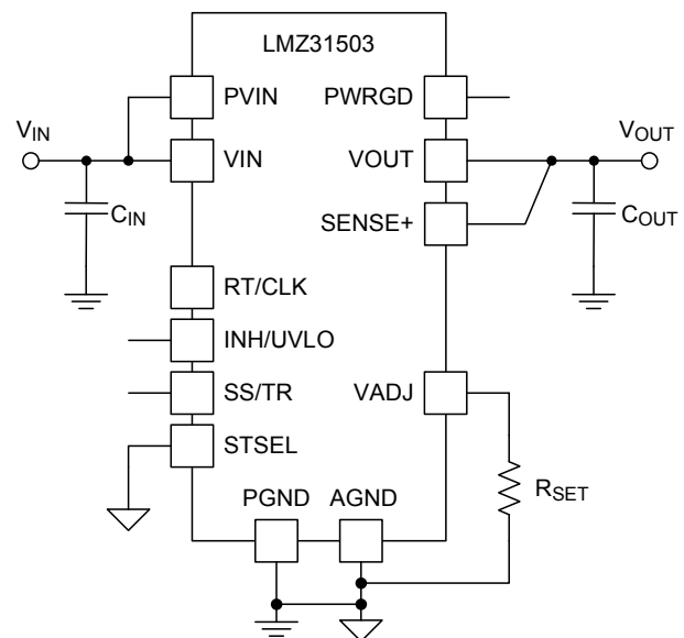
概略回路図
