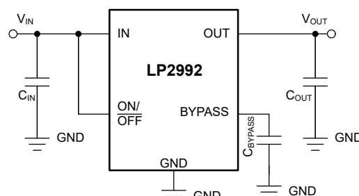
代表的なアプリケーション回路
