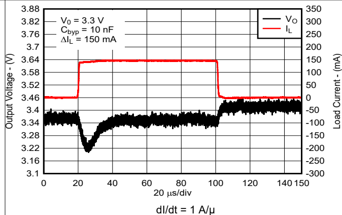
図 7-4. Load Transient for New Chip
