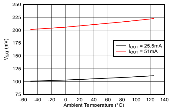
図 6-3. V SAT と温度との関係
