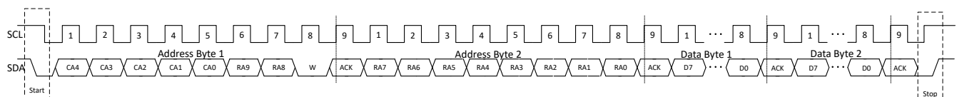
図 7-21. I 2 C 書き込みタイミング
