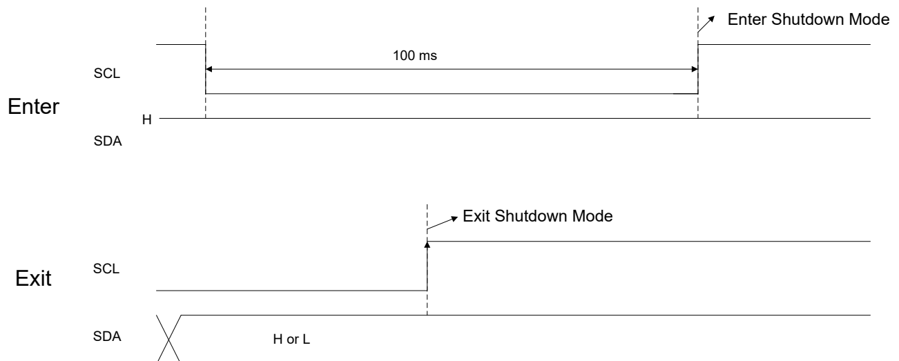
図 7-11. シャットダウンモード方式ペア 2 の開始と終了
