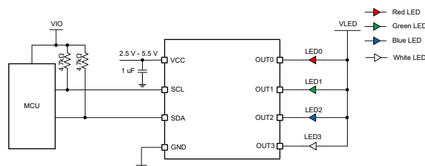
LP5814 の概略回路図
