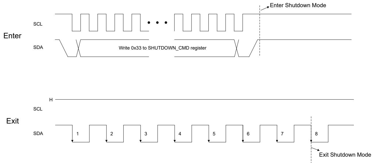
図 7-10. シャットダウンモード方式ペア 1 の開始と終了
