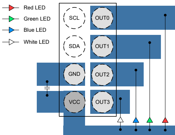
図 8-8. LP5814 YCH パッケージのレイアウト例
