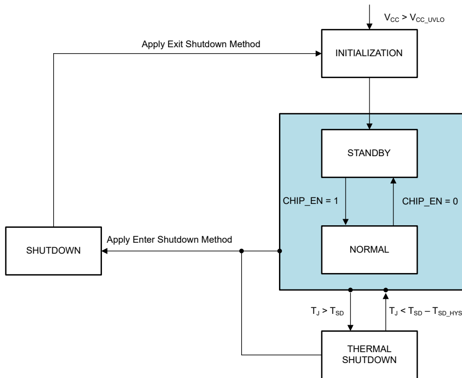
図 7-4. 機能モード
