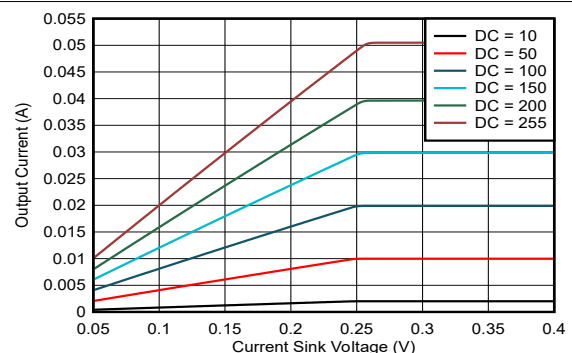
図 6-3. 電流シンク電圧と電流との関係 (MC = 1、 V_{CC} = 2.5\text{V} )
