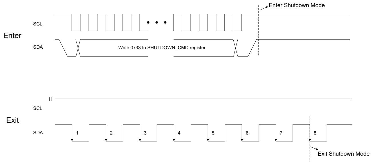
図 7-5. シャットダウンモード方式ペア 1 の開始と終了
