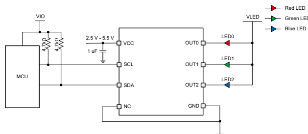
LP5817 の概略回路図
