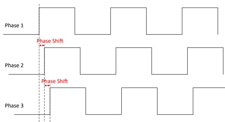
図 7-4. Phase Shift
