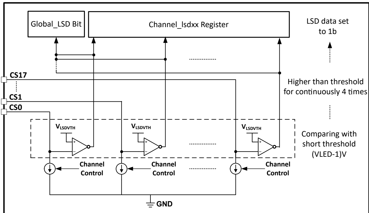
図 7-12. LSD Circuit
