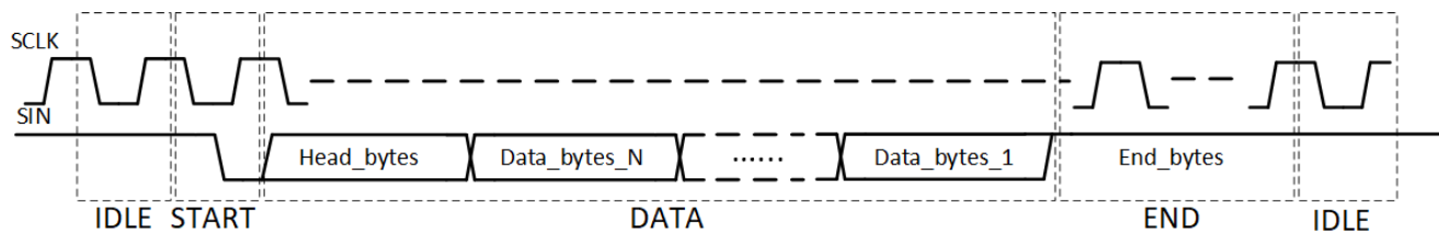
☒ 7-17. CCSI Frame
