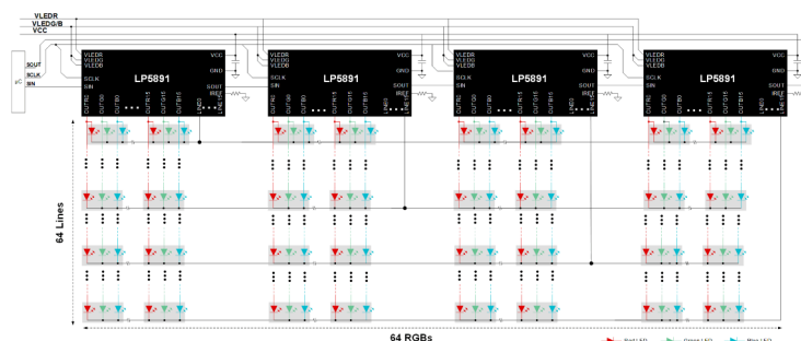
LP5891 4 デバイス・スタック接続
