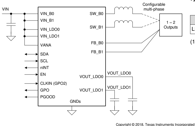
概略回路図
