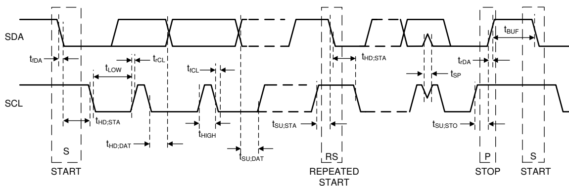
図 6-1. I 2 C-Compatible Timing
