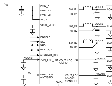
概略回路図
