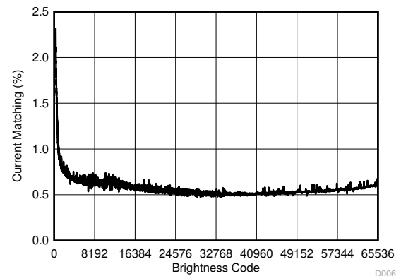
図 5-7. Current Matching
