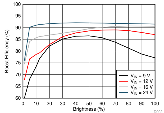
図 5-3. Boost Efficiency
