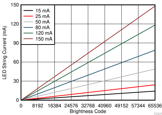
図 5-6. Current Linearity
