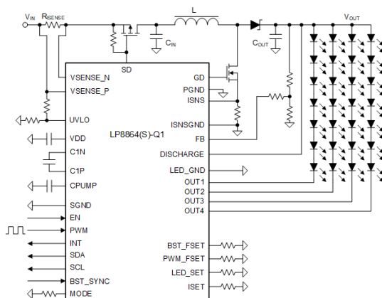
概略回路図
