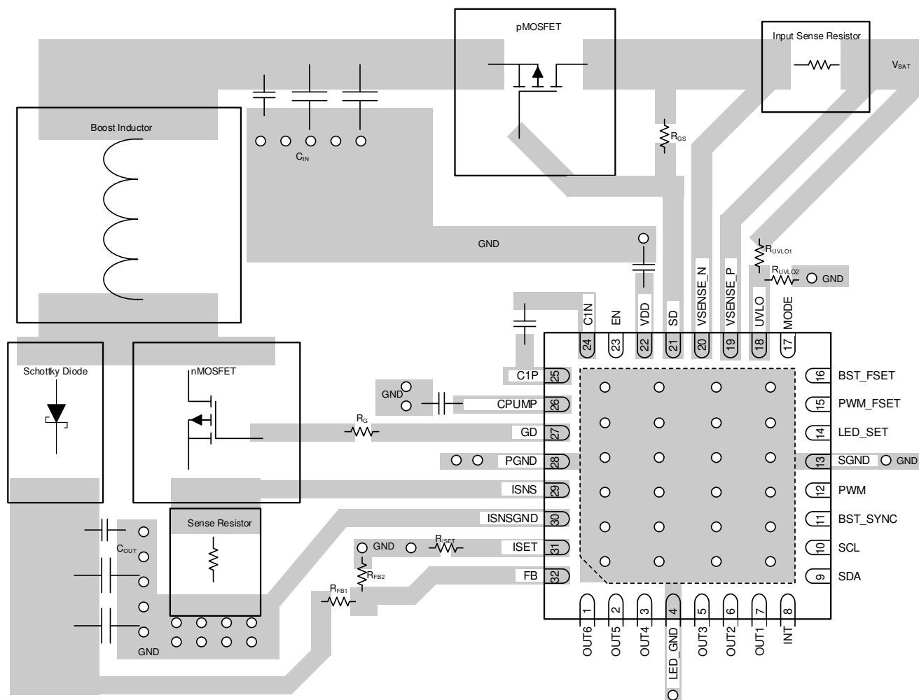
図 8-8. LP8866-Q1 Layout Guidelines
