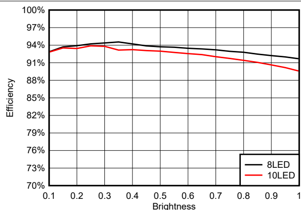
図 6-11. アナログ調光を使用する際の 1A の最大出力電流時の効率、 22μH インダクタ、昇圧トポロジ
