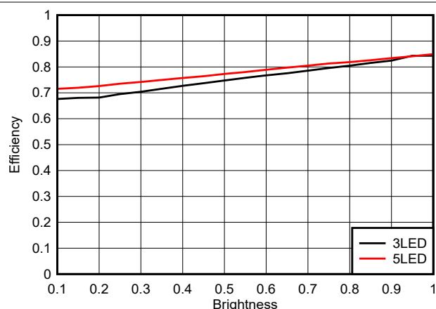
図 6-9. PWM 調光を使用する際の 1A の最大出力電流時の効率、 22μH インダクタ、昇降圧トポロジ
