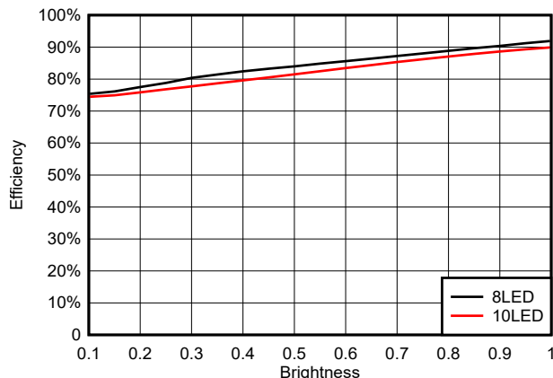
図 6-8. PWM 調光を使用する際の 1A の最大出力電流時の効率、 22μH インダクタ、昇圧トポロジ
