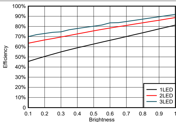
図 6-10. PWM 調光を使用する際の 3A の最大出力電流時の効率、 22μH インダクタ、降圧トポロジ
