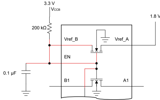
図 7-1. イネーブル ピンを V_{\text{ref\_B}} に直接接続およびバイアス抵抗を介して V_{\text{CCB}} に接続
