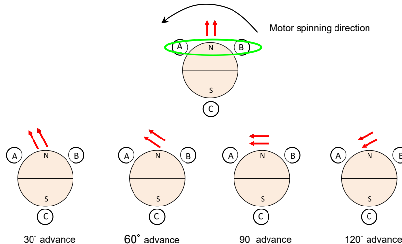
図 6-36. IPD アドバンス角度
