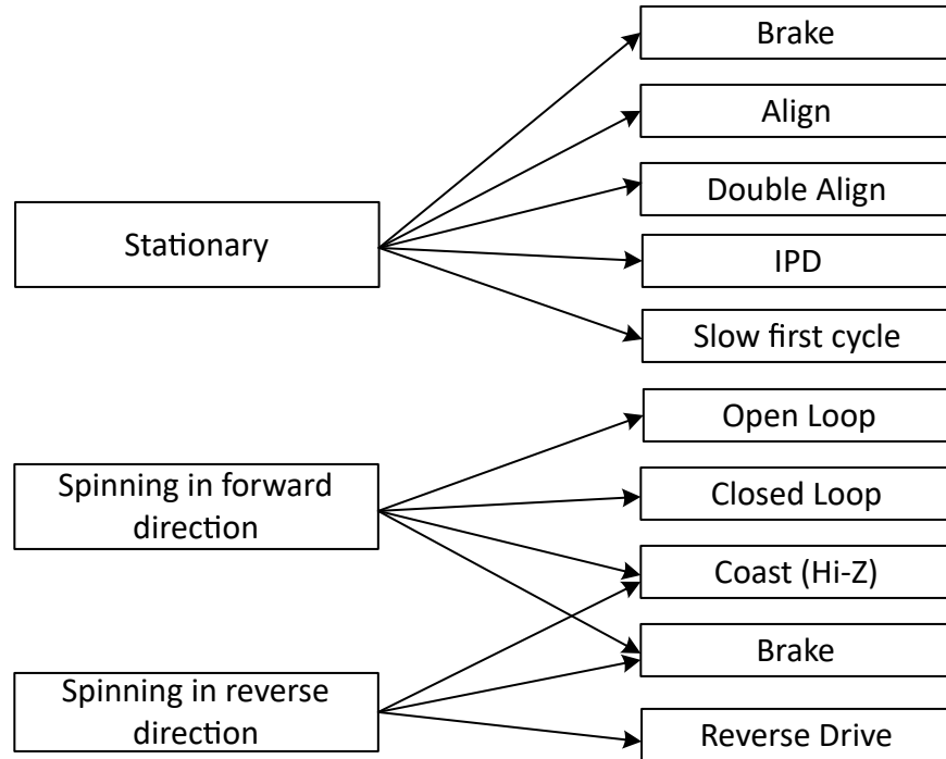
図 6-29. 異なる初期条件でのモータの起動
