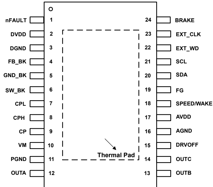
図 4-3. MCF8315D 24 ピン HTSSOP (露出サーマルパッド付き) 上面図
