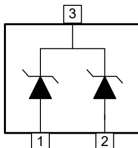
機能図
