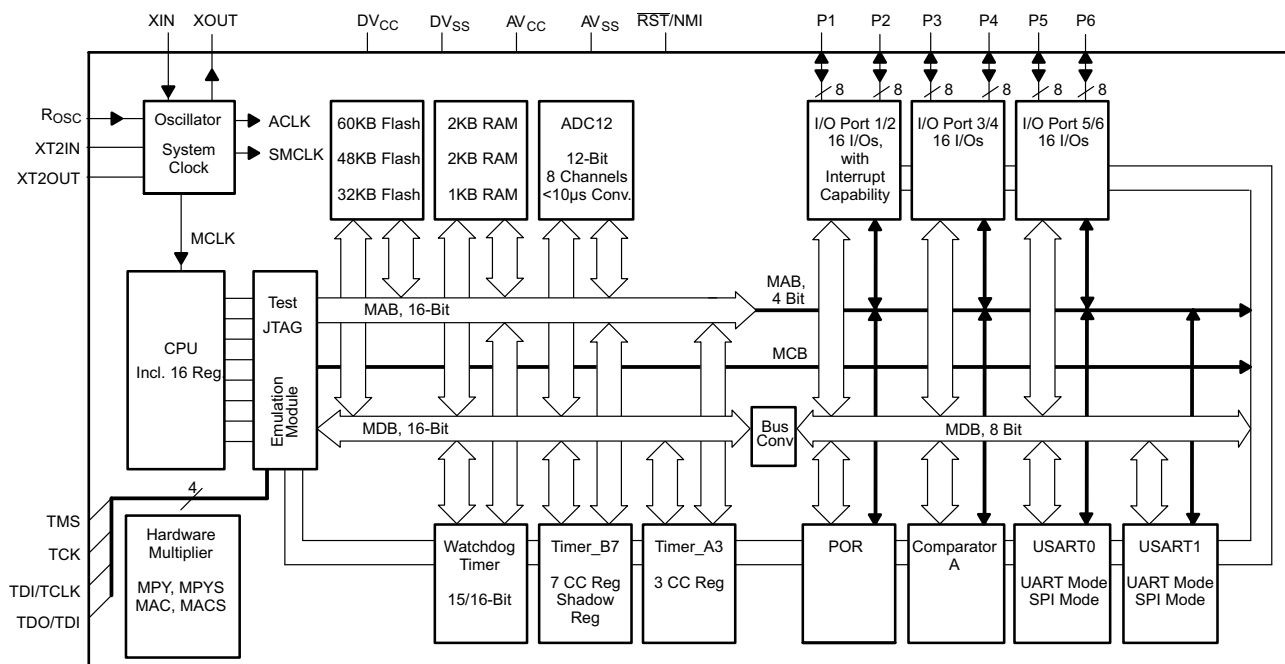
図 1-2. MSP430F14xの機能ブロック図
