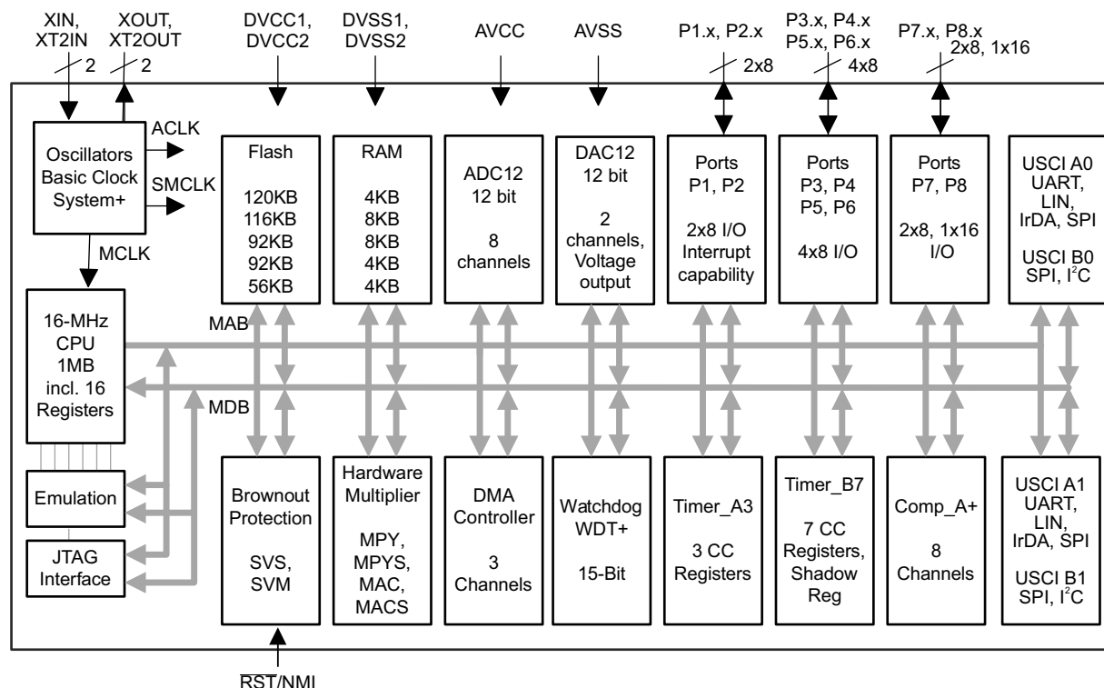
図 4-3. MSP430F261x 機能ブロック図、PN または ZCA パッケージ
