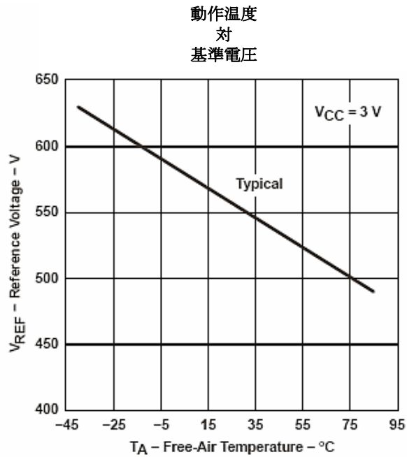
図 6. 動作温度 対 V_{REF} ( V_{CC} = 3\text{ V} )
