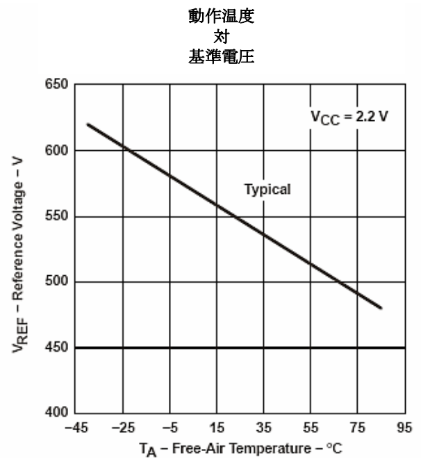
図 7. 動作温度 対 V_{REF} ( V_{CC} = 2.2\text{ V} )
