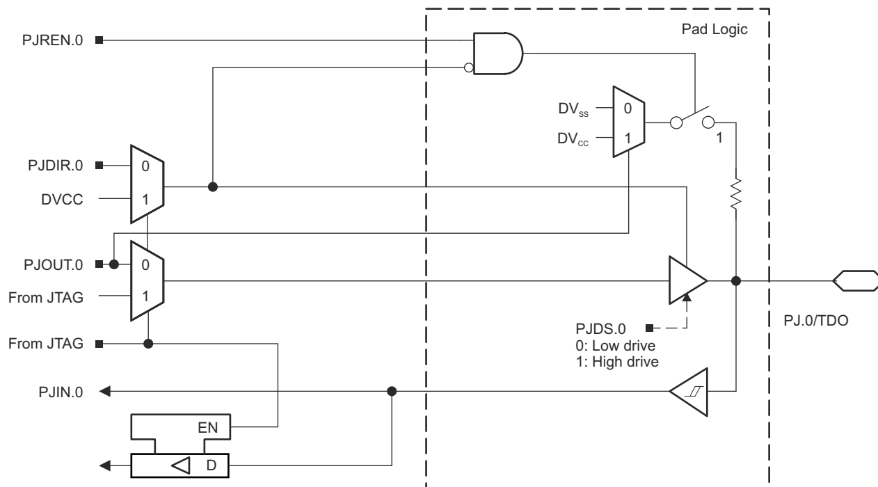
図 9-13. Port PJ (PJ.0) Diagram
