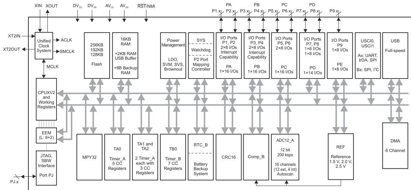
図 4-2. 機能ブロック図 – MSP430F5635, MSP430F5634, MSP430F5633
