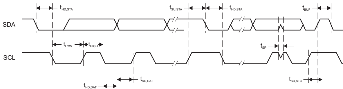
图 5-15. I 2 C Mode Timing
