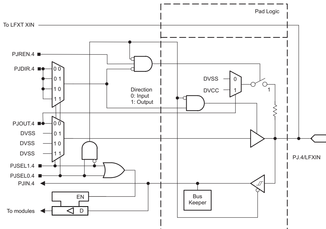
図 6-6. Port PJ (PJ.4) Diagram
