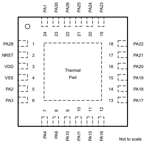
図 6-5. 24 ピン RGE (VQFN) (上面図)
