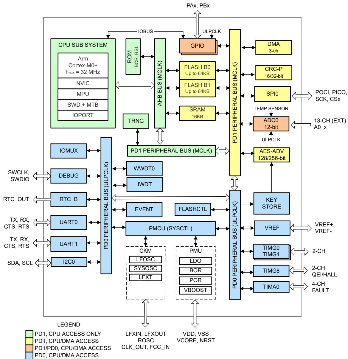
図 4-1. MSPM0L111x-Q1 の機能ブロック図
