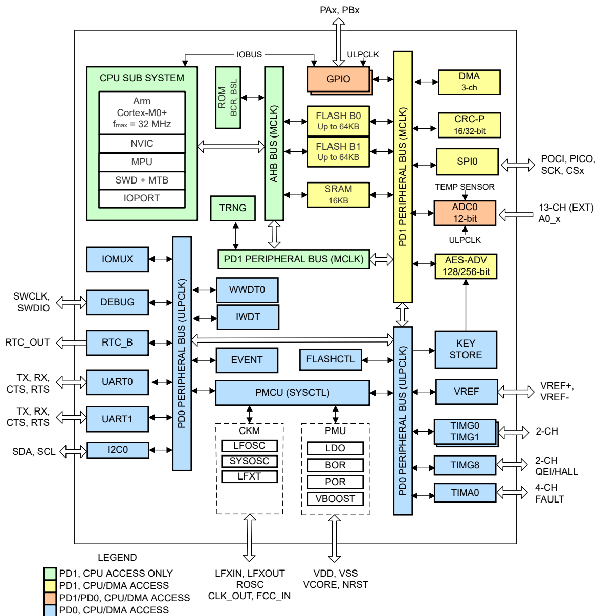
図 8-1. MSPM0L111x-Q1 の機能ブロック図
