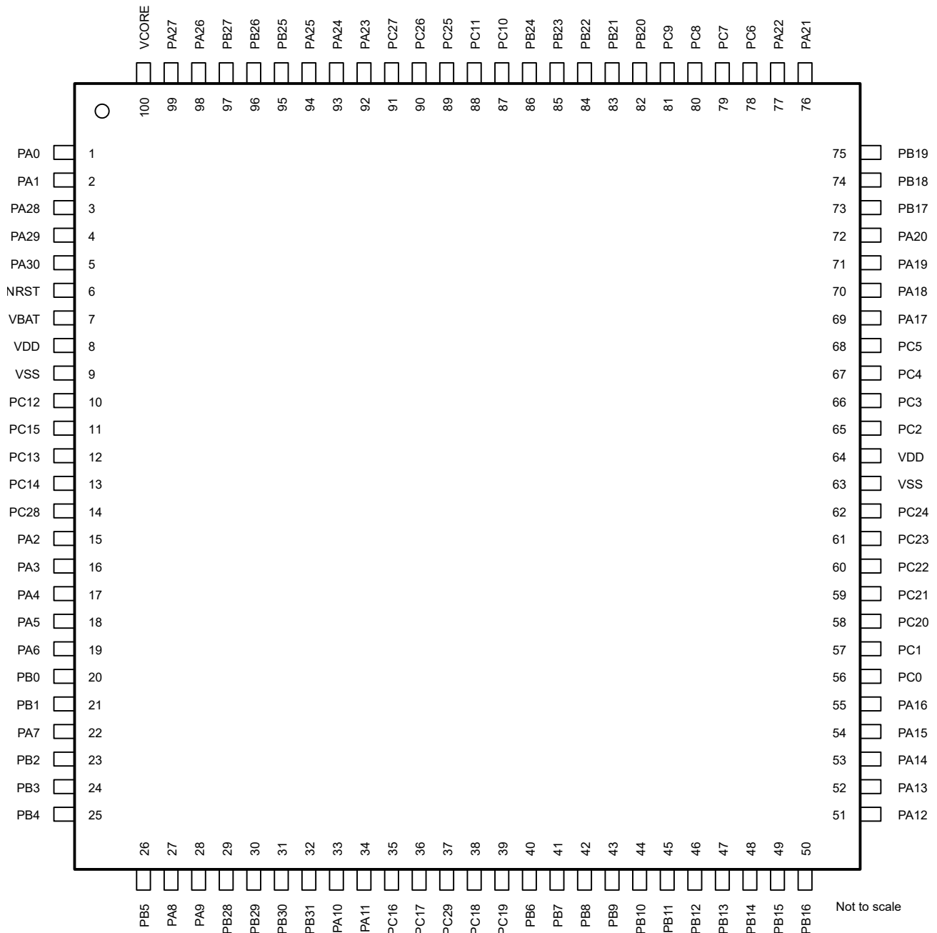
図 6-2. 100 ピン PFA (14mm × 14mm) (0.4mm ピッチ) および PZ (16mm × 16mm) (0.5mm ピッチ) (LQFP) パッケージ図 (上面図)
