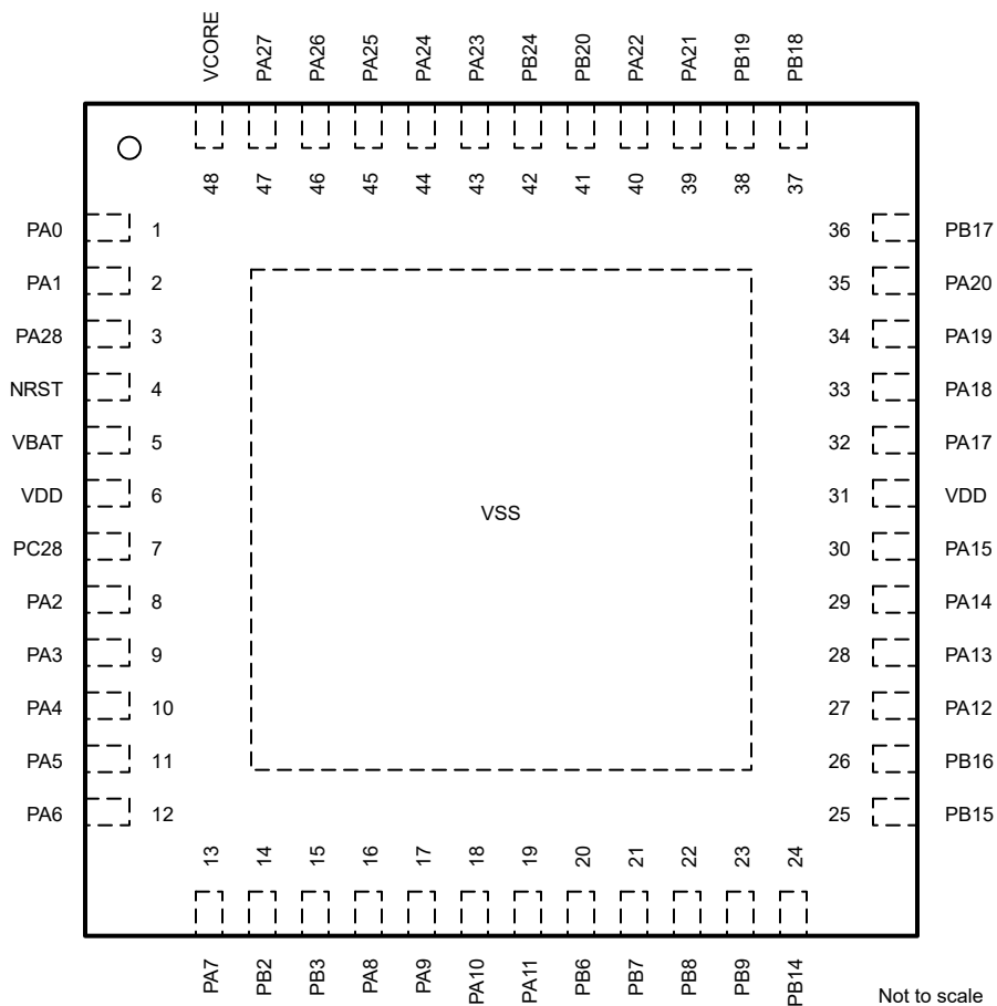
図 6-5. 48 ピン RGZ (7mm x 7mm) (0.5mm ピッチ) (VQFN) パッケージ図 (上面図)
