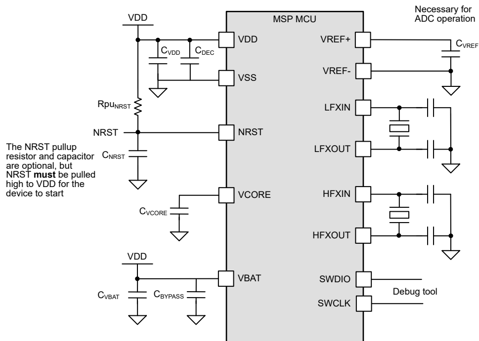
図 9-1. 基本アプリケーションの回路図
