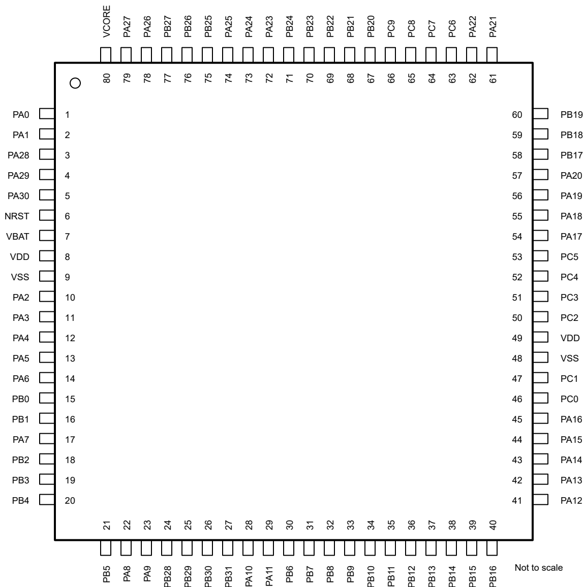
図 6-3. 80 ピン PN (14mm x 14mm) (0.5mm ピッチ) (LQFP) パッケージ (上面図)
