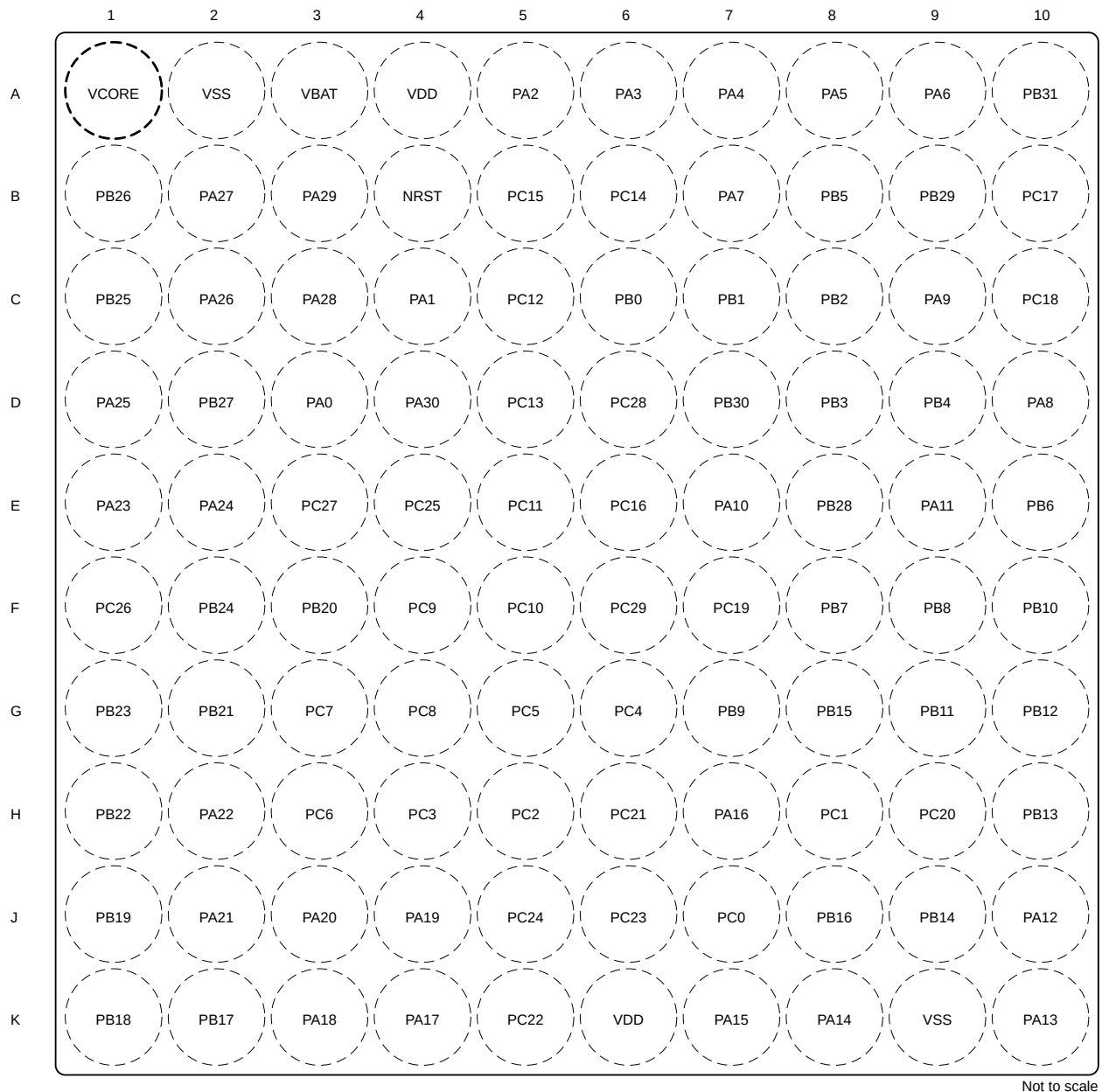
図 6-1. 100 ピン ZAW (9mm x 9mm) (0.8mm ピッチ) (NFBGA) パッケージ図 (上面図)
