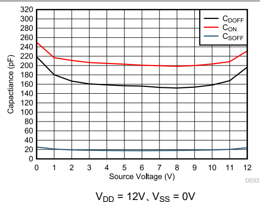
図 6-26. 容量とソース電圧またはドレイン電圧との関係
