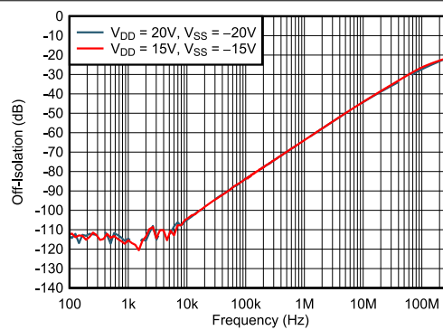
図 6-18. オフ絶縁と周波数との関係
