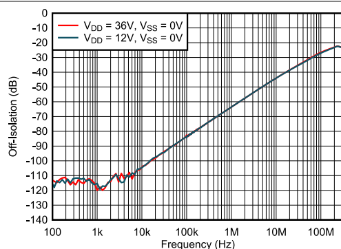
図 6-19. オフ絶縁と周波数との関係
