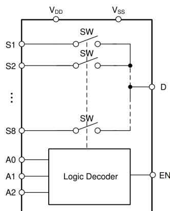
MUX708-Q1 ブロック図
