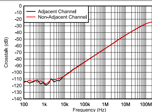
図 6-20. クロストークと周波数との関係
