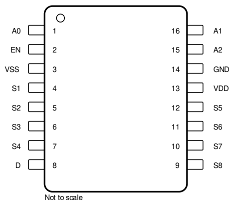
図 5-1. MUX708-Q1 : PW パッケージ 16 ピン TSSOP 図 5-2. MUX708-Q1 : RUM パッケージ 16 ピン WQFN 上面図
