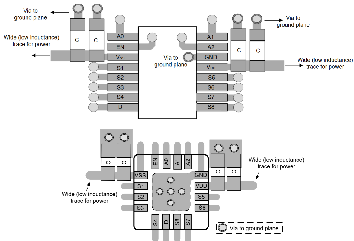
図 9-5. MUX708-Q1 のレイアウト例
