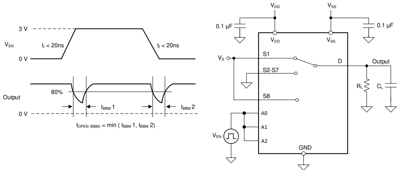
図 7-6. ブレイク ビフォー メイク遅延測定時の構成
