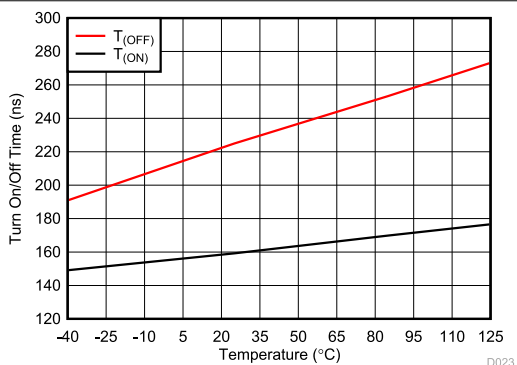
図 6-17. T_{\text{ON}} および T_{\text{OFF}} と温度との関係 V_{\text{DD}} = 44\text{V} , V_{\text{SS}} = 0\text{V}
