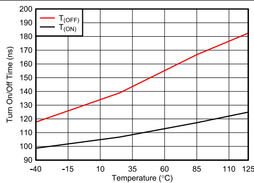
図 6-16. T_{\text{ON}} および T_{\text{OFF}} と温度との関係 V_{\text{DD}} = 15\text{V} , V_{\text{SS}} = -15\text{V}
