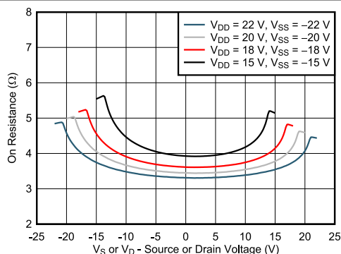
図 6-1. オン抵抗とソースまたはドレイン電圧との関係 – デュアル電源
