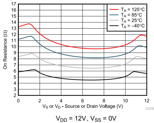
図 6-7. オン抵抗と温度との関係
