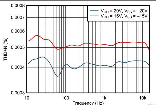
図 6-21. THD+N と周波数との関係 (デュアル電源)
