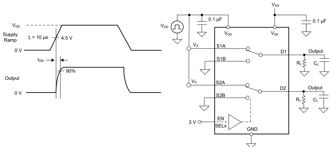
図 7-7. t_{ON}(V_{DD}) 時間の測定に使用する構成
