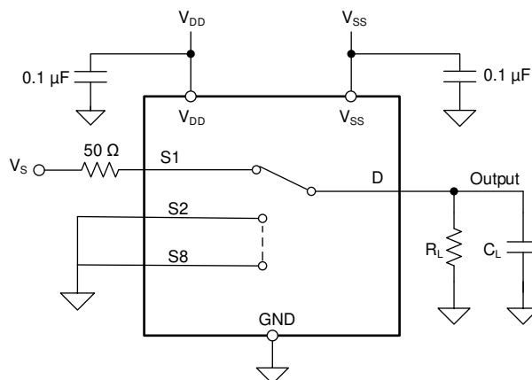
図 7-8. 伝搬遅延測定時の構成
