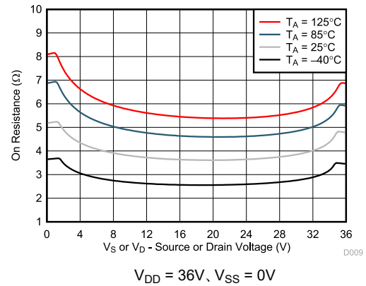
図 6-8. オン抵抗と温度との関係
