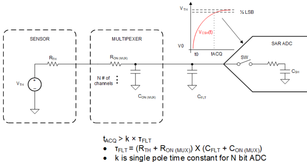
図 9-2. 逐次比較型 ADC の駆動
