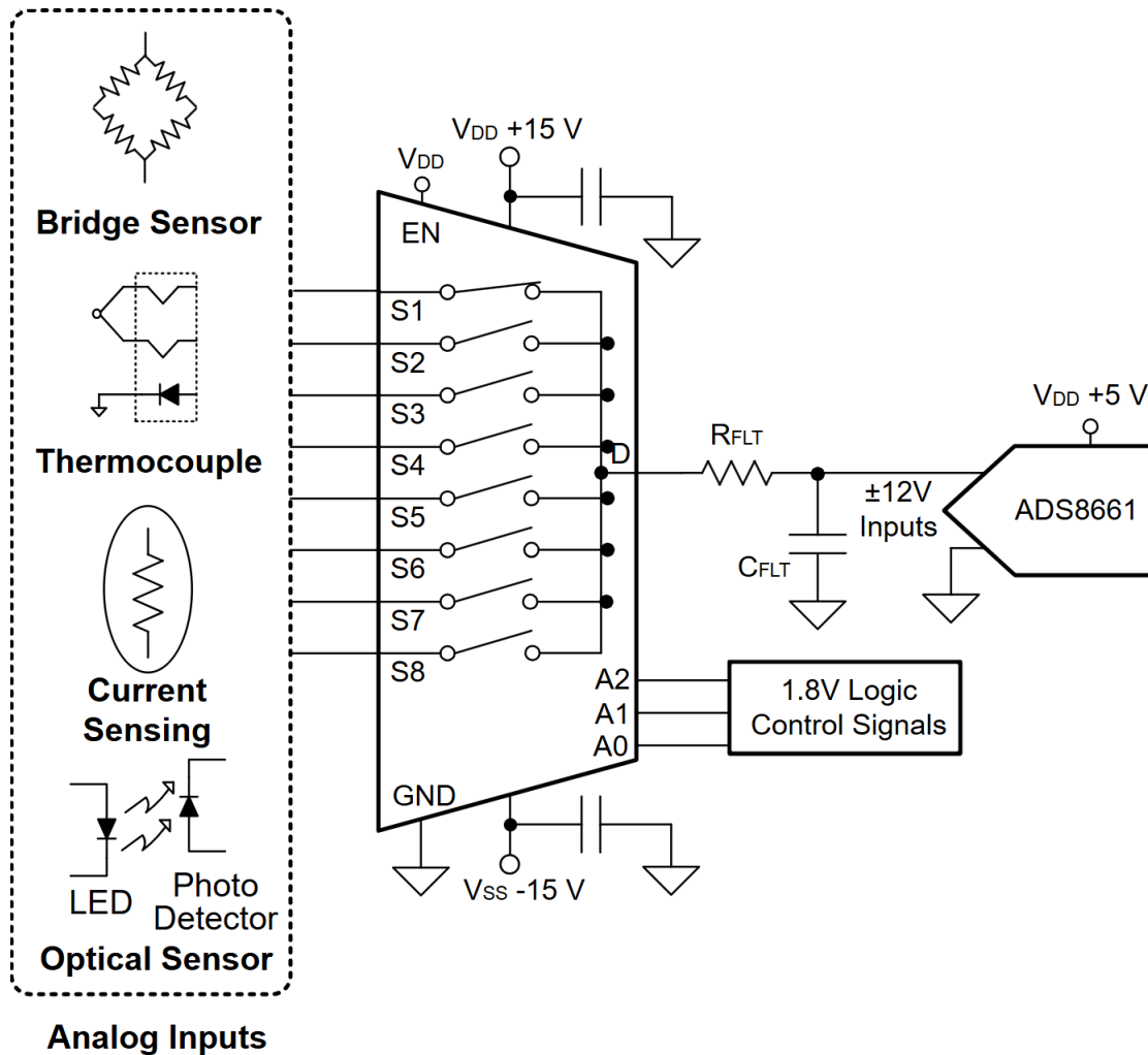
図 9-1. 多重化されたデータ アキュイジション フロント エンド
