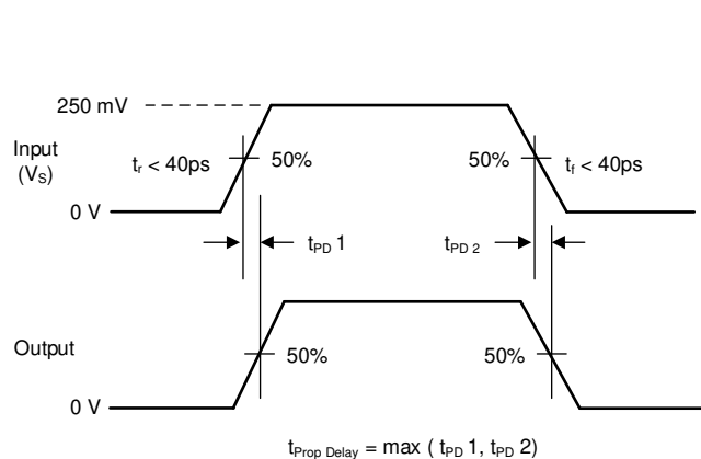
図 7-8. 伝搬遅延測定時の構成
