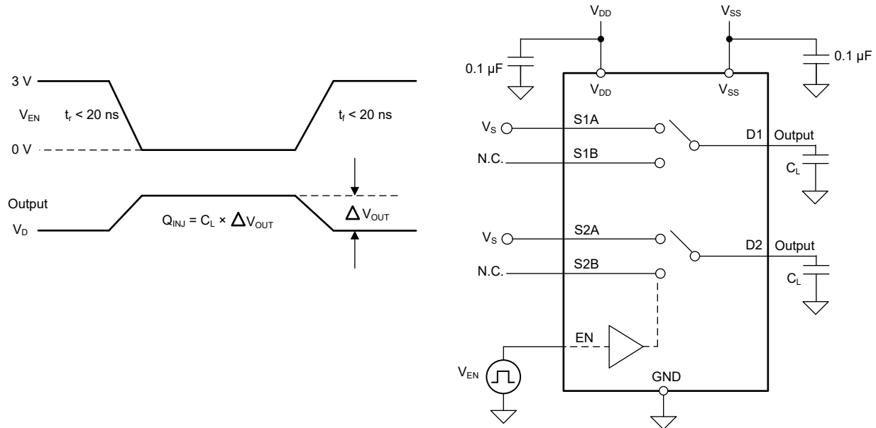
図 7-9. 電荷注入測定時の設定
