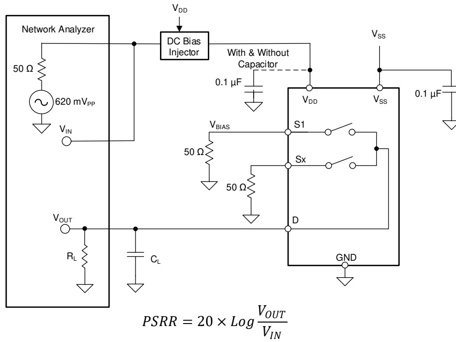
図 7-14. ACPSRR 測定のセットアップ
