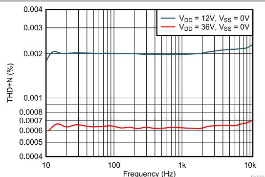
図 6-22. THD+N と周波数との関係 (単一電源)
