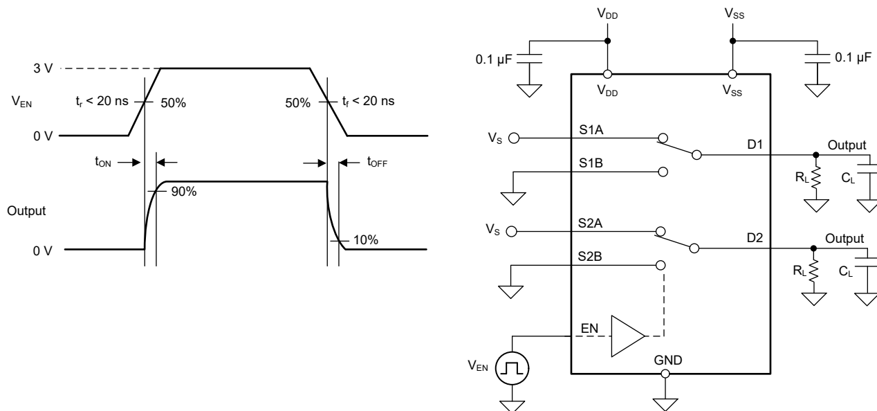
図 7-5. ターンオンおよびターンオフ時間の測定に使用する構成
