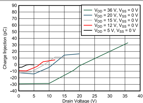
図 6-13. チャージ インジェクションとドレイン電圧との関係 – 単一電源
