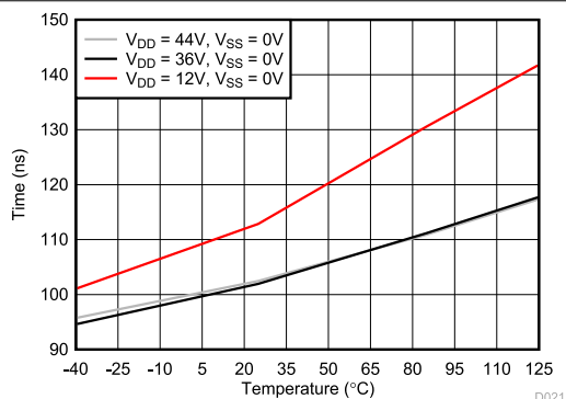
図 6-15. T_{\text{TRANSITION}} と温度との関係
