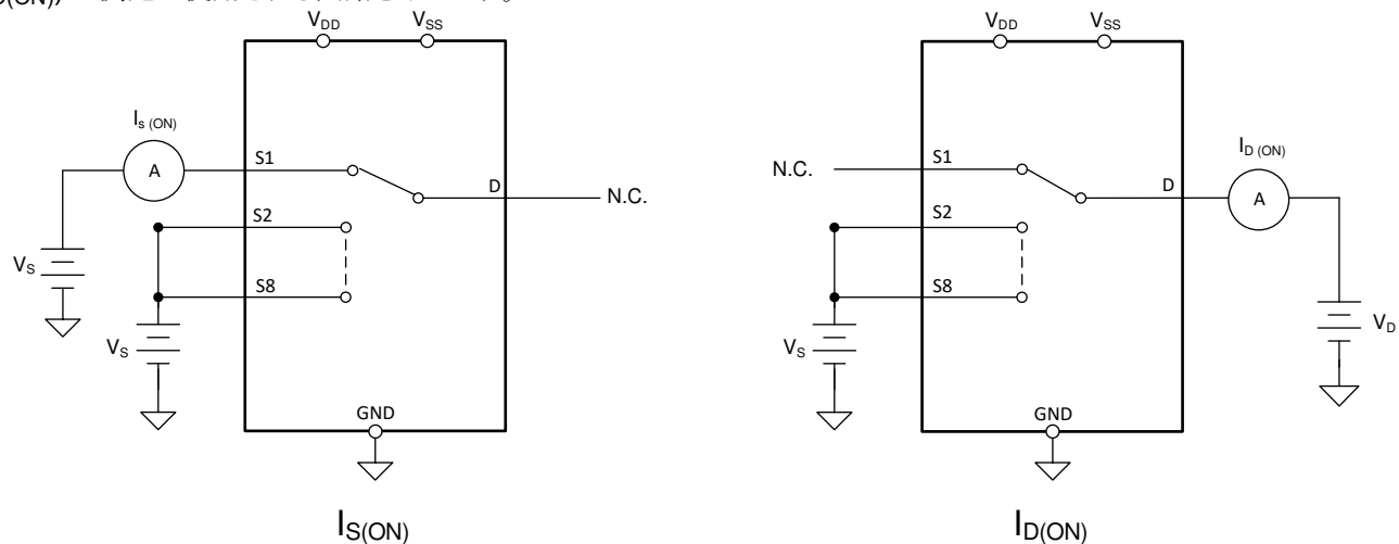
図 7-3. オン リーク測定時の構成
