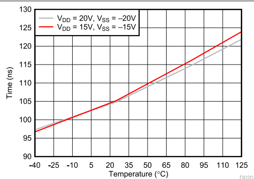
図 6-14. T_{\text{TRANSITION}} と温度との関係
