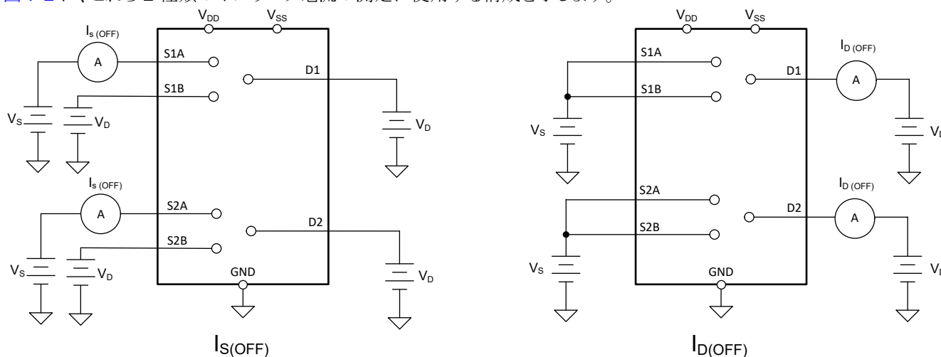
図 7-2. オフ リーク測定時の構成
