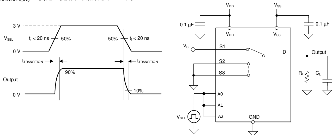
図 7-4. 遷移時間測定時の構成
