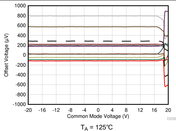
図 5-25. オフセット電圧と同相電圧との関係 (新しいダイ)
