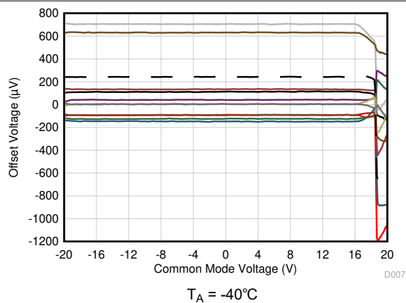
図 5-24. オフセット電圧と同相電圧との関係 (遷移領域) (新しいダイ)
