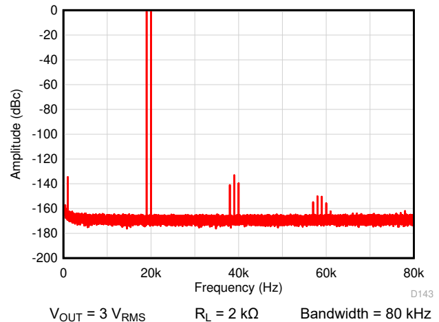
FIG 6-14. FFT, CCIF Input (19 kHz + 20 kHz)
