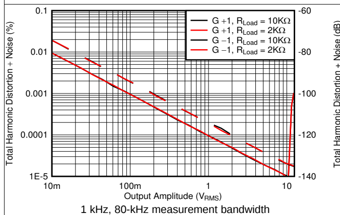
图 11. THD+N vs Output Amplitude
