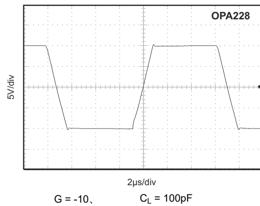
図 6-32. 大信号ステップ応答
