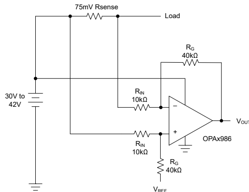
図 7-4. 36V バッテリー ハイサイド電流センス
