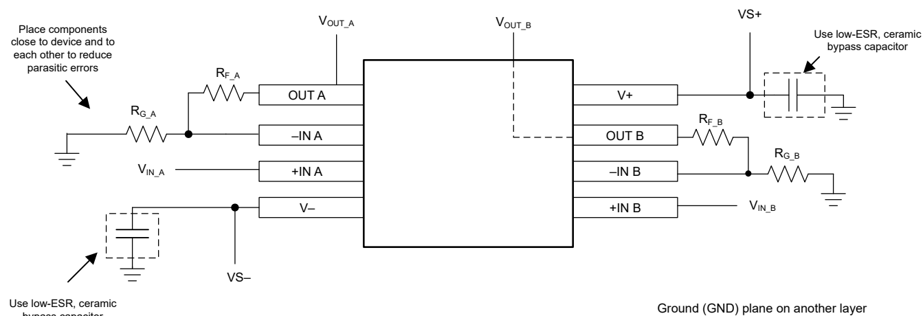
図 7-6. VSSOP-8 パッケージの非反転構成の基板レイアウト
