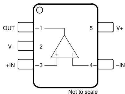
図 4-1. OPA986 DBV パッケージ、5 ピン SOT-23 (上面図)
