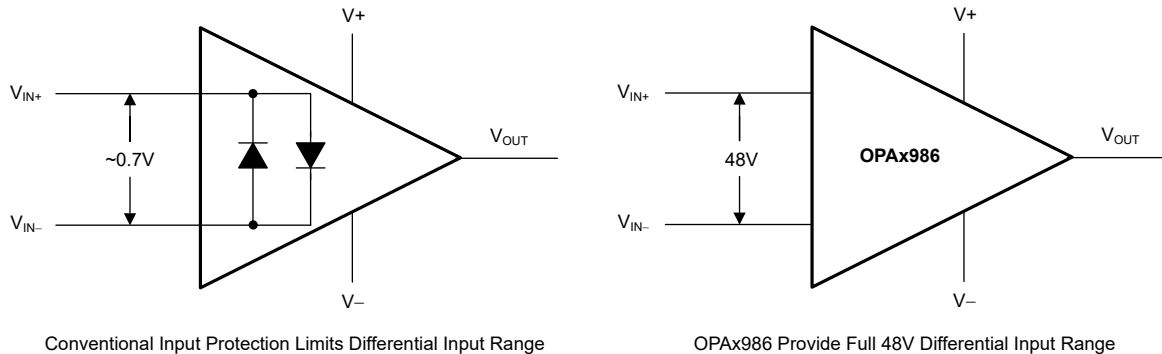
図 6-1. OPAx986 の入力保護機能は、差動入力能力を制限しない
