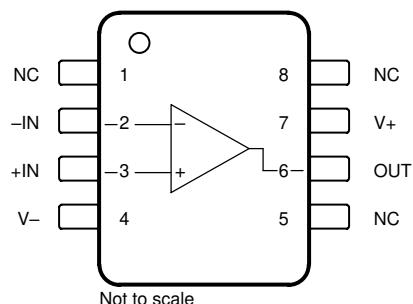
図 4-2. OPA986 D パッケージ、8 ピン SOIC (上面図)
