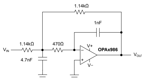
図 7-1.2 次、マルチ フィードバック ベッセル応答ローパス フィルタ
