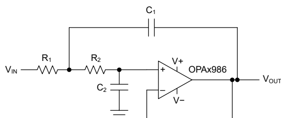
サレンキー型ローパス フィルタ
