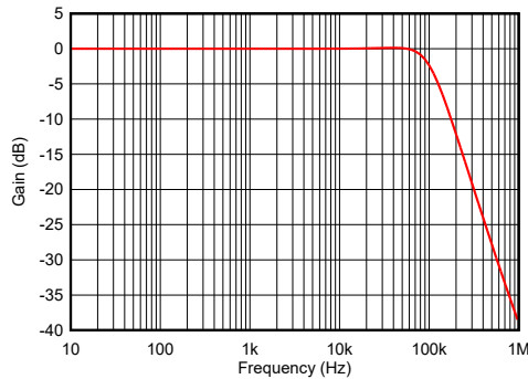
図 7-2. 全周波数帯域ゲイン応答
