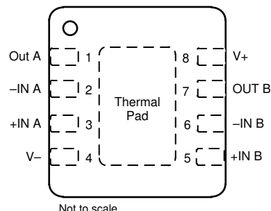
図 4-4. OPA2596 DSG (プレビュー) パッケージ、8 ピン WSON (上面図)
