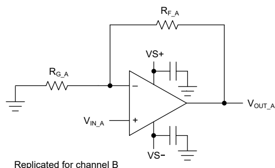
図 7-5. 非反転構成の回路図
