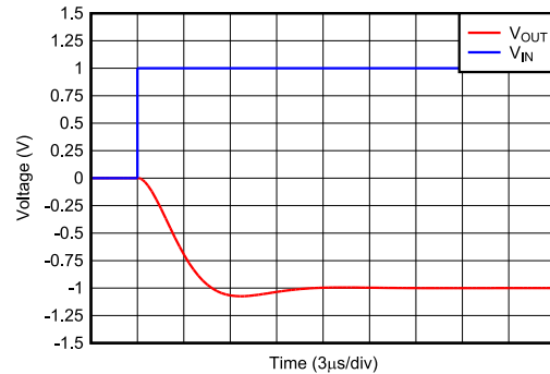
図 7-3. 過渡応答
