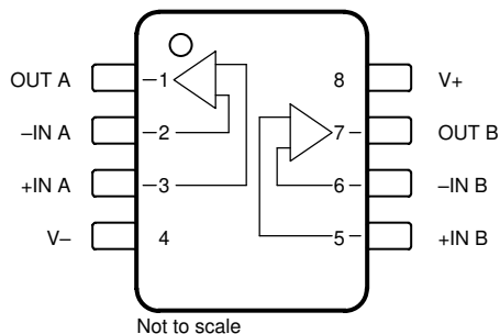
図 4-3. OPA2986 D (プレビュー) パッケージ、8 ピン SOIC および DGK (プレビュー) パッケージ、8 ピン
