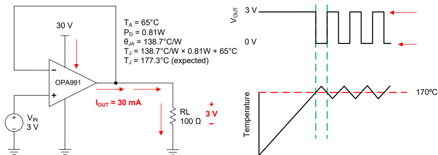
FIG 7-4. Thermal Protection
