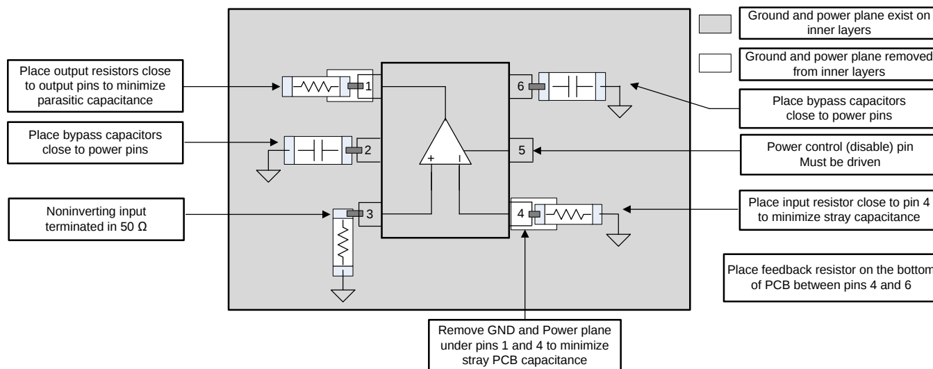
图 40. Layout Example
