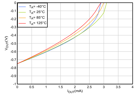
図 5-16. 出力電圧と出力電流との関係 ( V_S = 1.5\text{V} )
