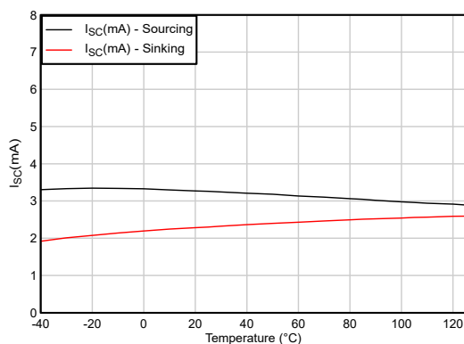
図 5-39. 短絡電流と温度との関係 ( V_S = 1.5\text{V} )
