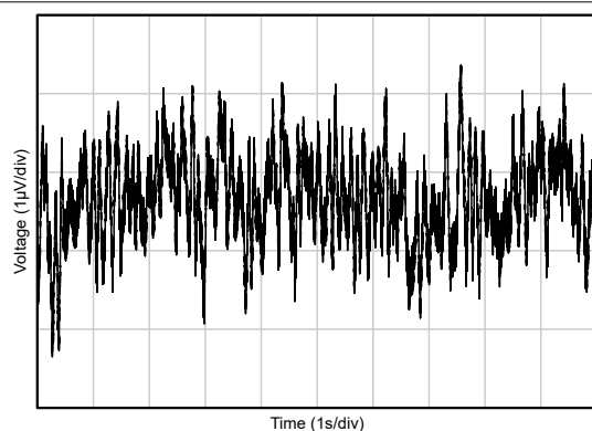
図 5-23. 時間領域での 0.1Hz~10Hz の電圧ノイズ
