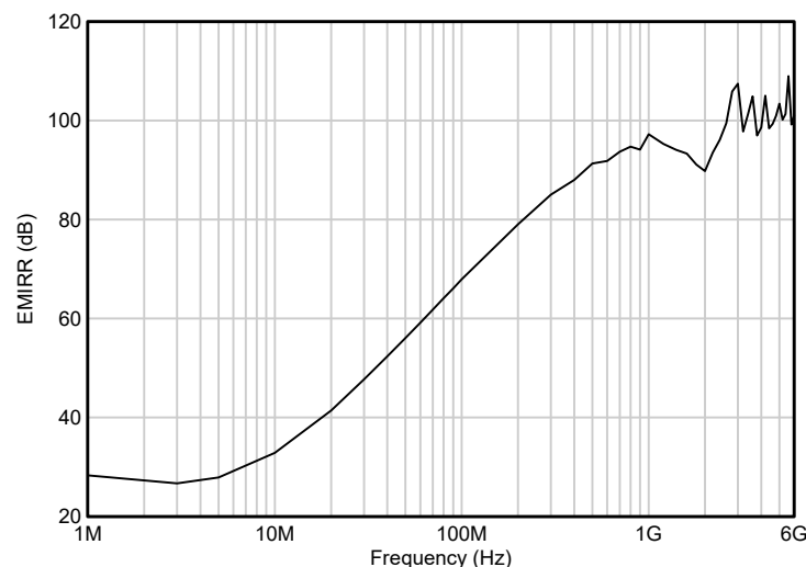
図 6-4. EMIRR テスト
