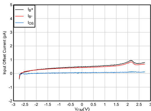
図 5-9. I_B および I_{OS} と同相電圧との関係
