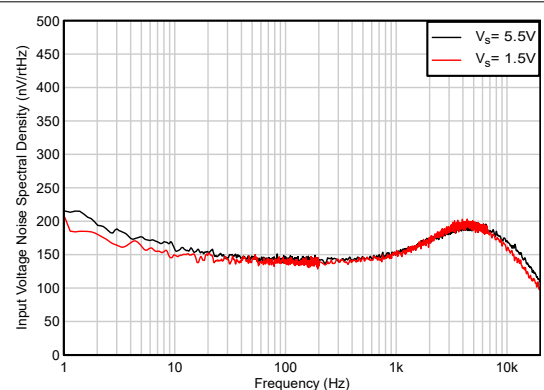
図 5-24. 入力電圧ノイズ スペクトル密度
