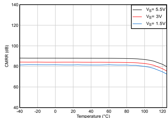
図 5-22. DC CMRR と温度との関係 ( (V_-) \geq V_{CM} \geq (V_+) - 0.7\text{V} )
