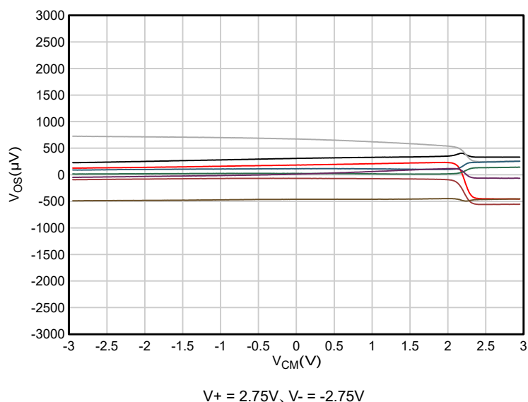
図 6-1. オフセット電圧と同相電圧との関係
