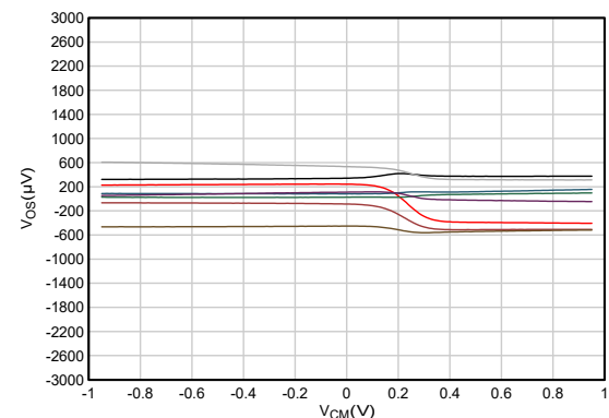
図 5-6. オフセット電圧と同相モード ( V_S = 1.5\text{V} ) との関係
