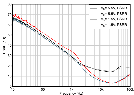
図 5-19. PSRR と周波数との関係
