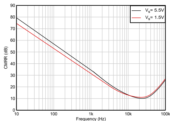
図 5-20. CMRR と周波数との関係
