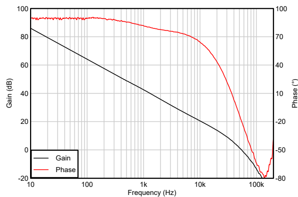
図 5-10. 開ループゲインおよび位相と周波数との関係
