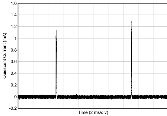
図 5-31. 過負荷時の静止電流
