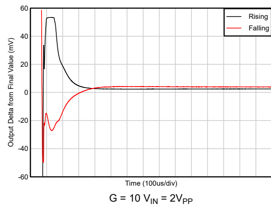
図 5-36. セットリング タイム
