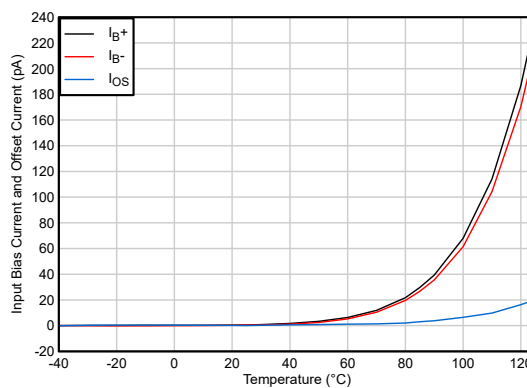
図 5-8. I_B および I_{OS} と温度との関係
