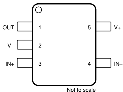
図 4-1. OPA371D DBV パッケージ 5 ピン SOT-23 上面図
