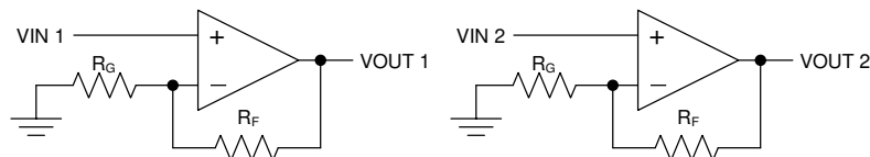
図 7-3. 回路図
