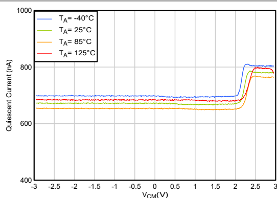
図 5-27. 静止電流と同相との関係
