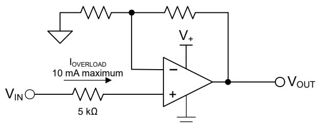
図 6-6. 入力電流保護
