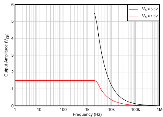
図 5-17. 最大出力電圧と周波数との関係
