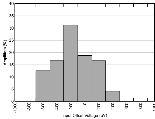
図 5-1. オフセット電圧のヒストグラム
