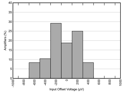
図 5-2. オフセット電圧ヒストグラム ( V_S = 1.5\text{V} )
