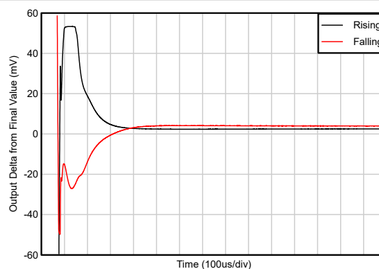
図 5-34. 大信号ステップ応答
