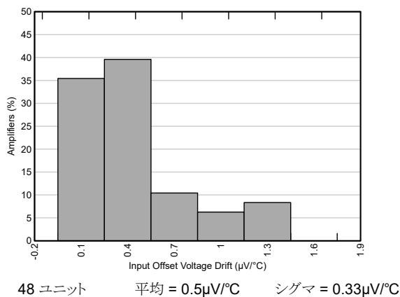
図 5-3. オフセット電圧ドリフト ヒストグラム ( 0^\circ\text{C} \sim 85^\circ\text{C} )
