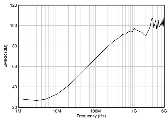
図 5-40. EMIRR と周波数との関係
