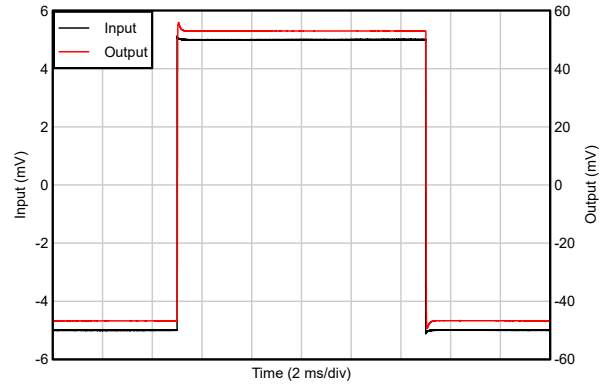
図 5-32. 小信号ステップ応答
