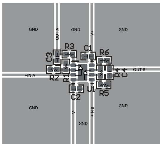
図 7-6. WSON-8 (DSG) パッケージのレイアウト例
