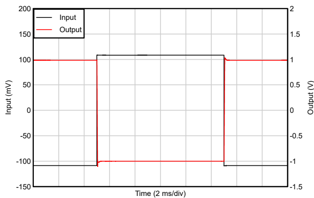
図 5-35. 大信号ステップ応答
