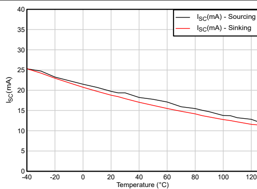
図 5-38. 短絡電流と温度との関係 ( V_S = 5.5\text{V} )
