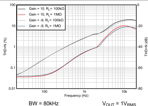
図 5-25. THD + N と周波数との関係
