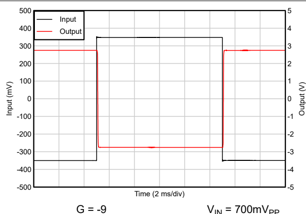
図 5-30. 過負荷回復
