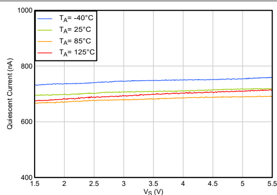
図 5-28. 静止電流と電源電圧との関係
