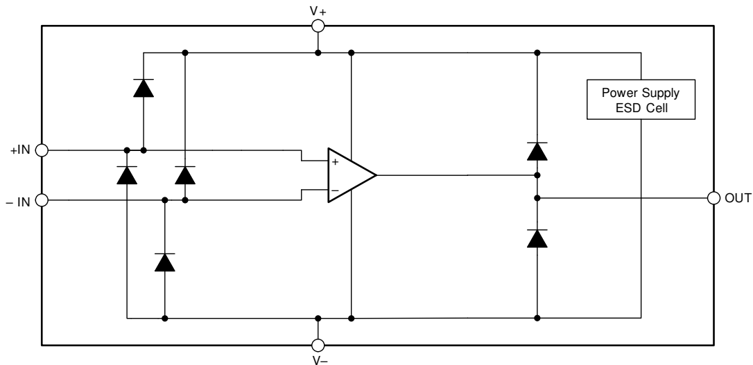
図 6-5. 内部 ESD 等価回路
