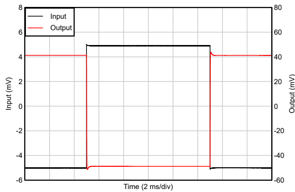
図 5-33. 小信号ステップ応答
