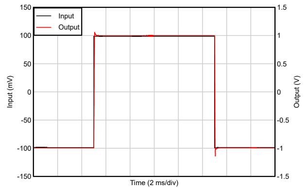
図 5-32. 小信号ステップ応答
