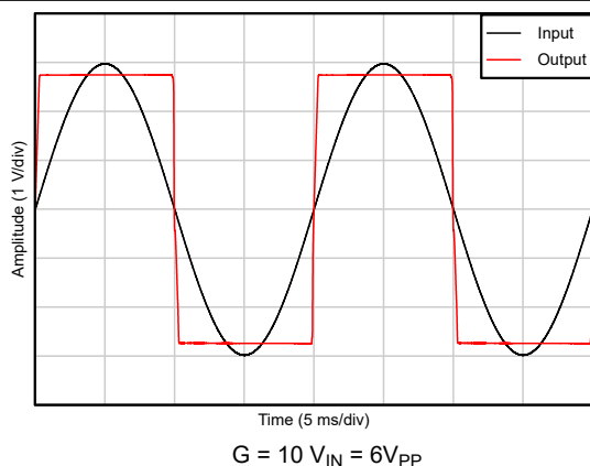
図 5-37. 位相反転が発生しない
