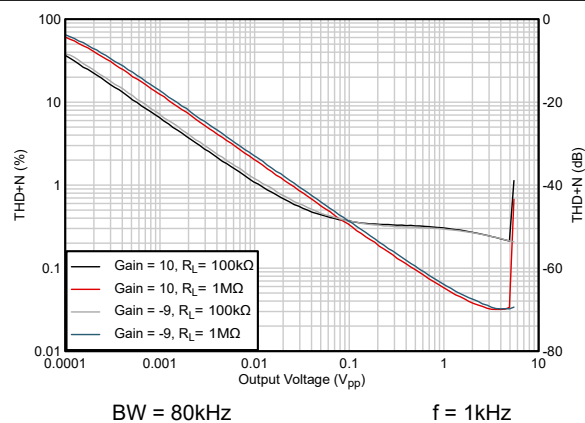
図 5-26. THD + N と振幅との関係
