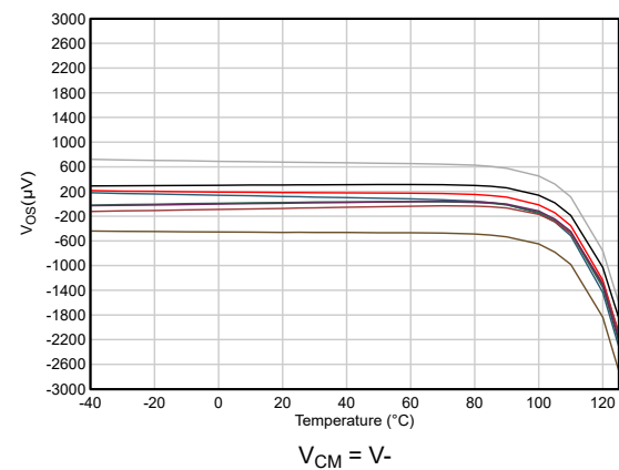
図 5-4. 入力オフセット電圧と温度との関係
