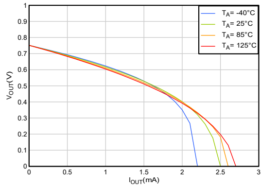
図 5-15. 出力電圧と出力電流との関係 ( V_S = 1.5\text{V} )
