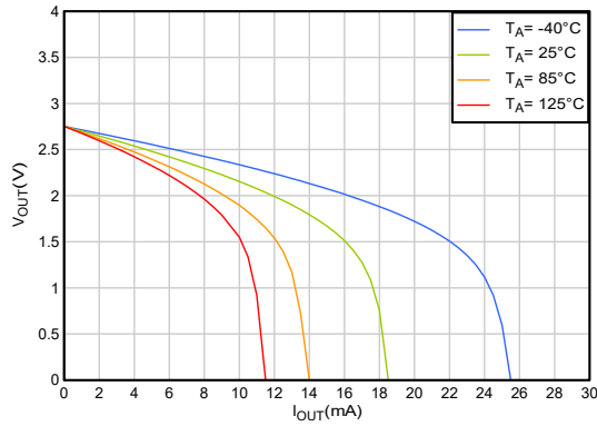
図 5-13. 出力電圧と出力電流との関係 (ソース)
