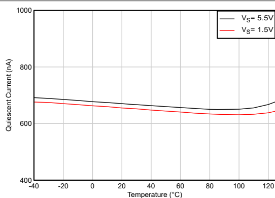
図 5-29. 静止電流と温度との関係
