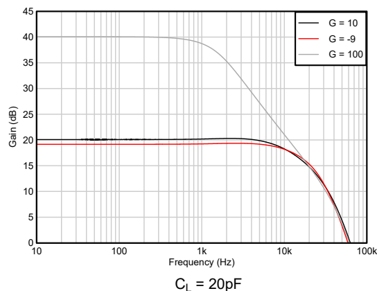
図 5-12. 閉ループゲインと周波数との関係
