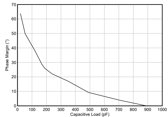
図 5-18. 位相マージンと容量性負荷との関係
