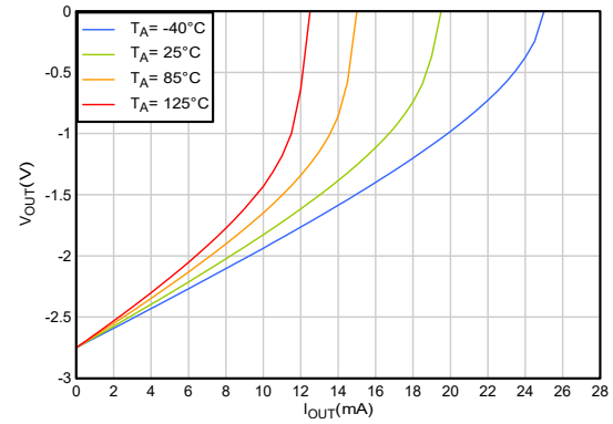
図 5-14. 出力電圧と出力電流との関係 (シンク)
