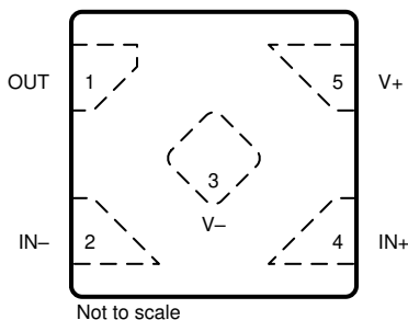
図 4-3. OPA371D DQN パッケージ 5 ピン SOT-5X3 上面図
