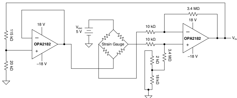
OPA2182 ブリッジ・センサ・アプリケーション
