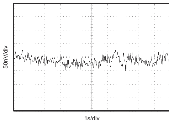
図 6-7. 入力ノイズ電圧と時間との関係
