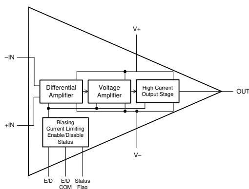
OPA455 のブロック図
