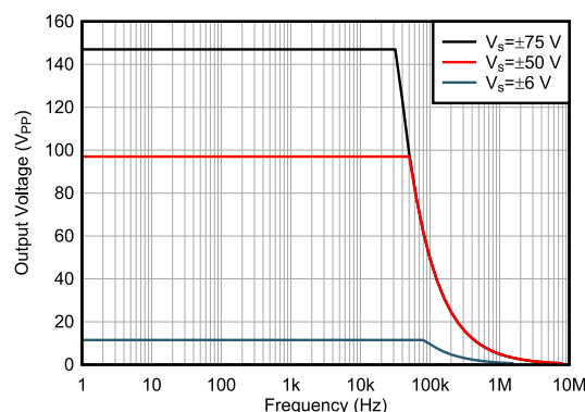
最大出力電圧と周波数との関係
