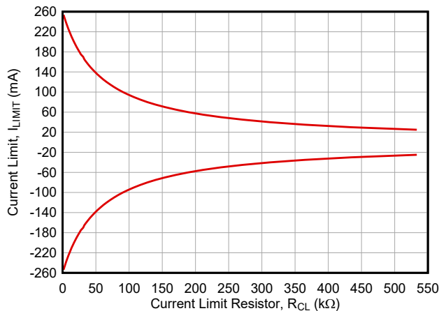
出力電流と電流制限抵抗の構成
