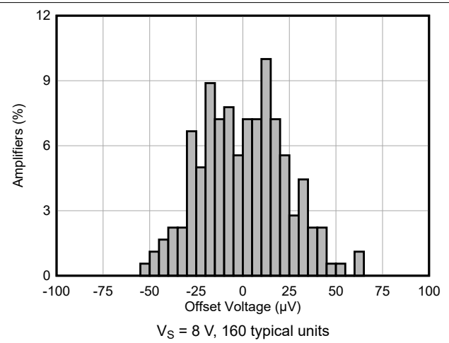
6-2. Input Offset Production Distribution
