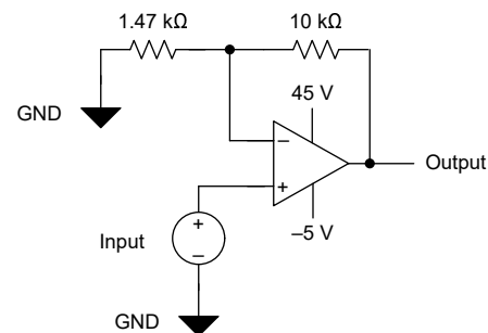
8 倍のゲイン構成の出力ドライバ
