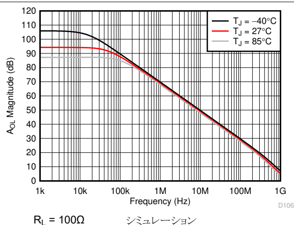
図 7-6. 開ループ ゲイン振幅と温度との関係
