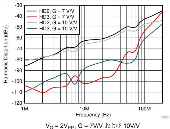
図 6-17. 高調波歪みとゲインにおける周波数との関係
