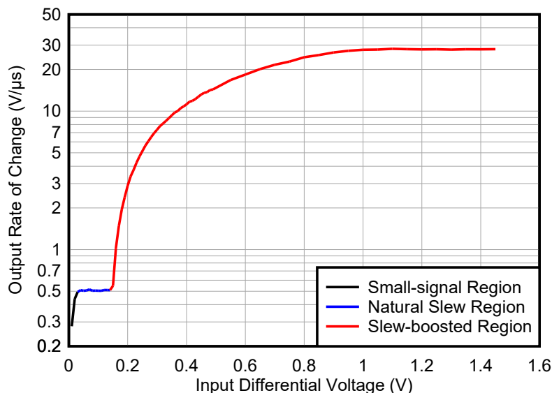
図 7-1. OPAx991-EP の出力変化率と入力差動電圧との関係
