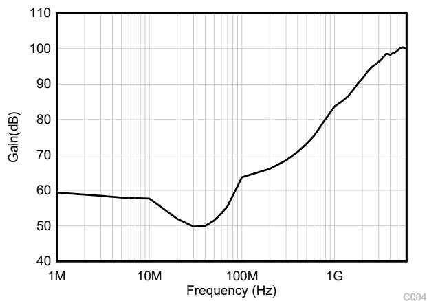
図 6-3. EMIRR テスト
