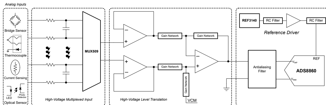
高電圧シグナル チェーンにおける OPAx991-EP
