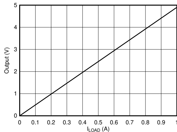
図 7-5. ローサイド、電流検出、伝達関数
