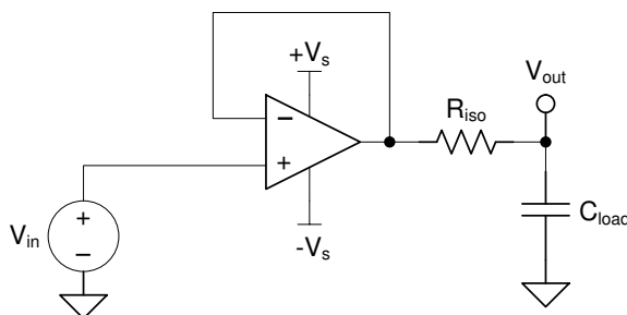
図 6-7. OPAx991-EP により容量性負荷の駆動能力を拡張
