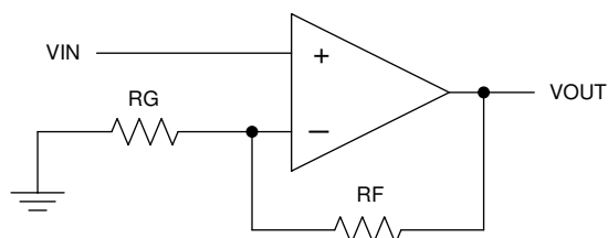
図 7-6. 回路図
