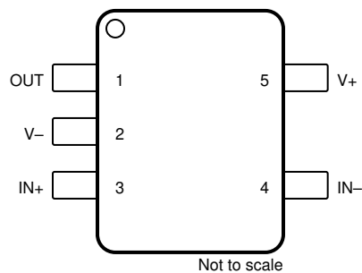
図 4-1. OPA991-EP DBV パッケージ 5 ピン SOT-23 (上面図)
