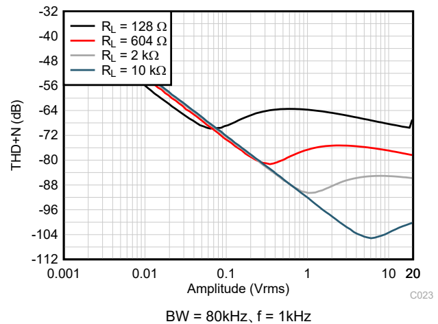
図 5-22. THD+N と出力振幅との関係
