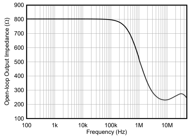
図 5-26. 開ループ出力インピーダンスと周波数との関係
