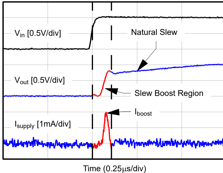
図 7-2. OPAx991-EP の大信号ステップ応答特性
