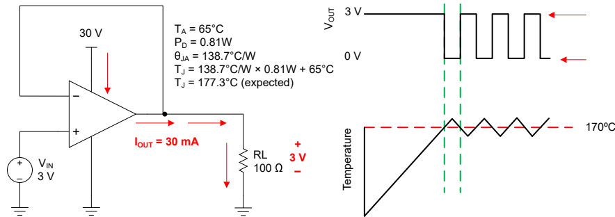
図 6-4. 過熱保護
