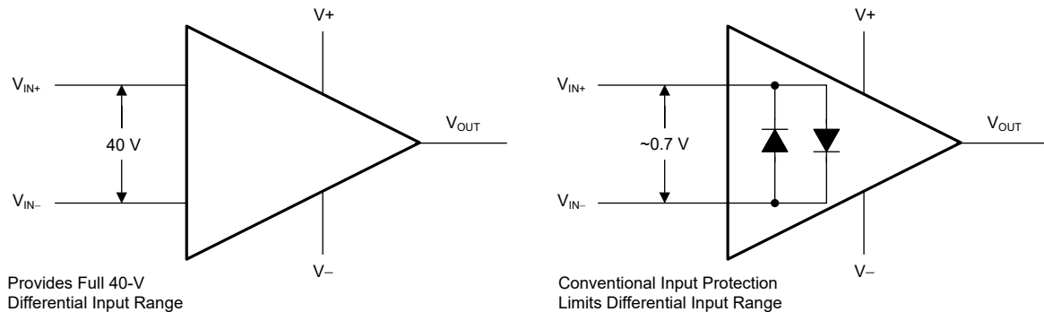
図 6-1. OPAx991-EP の入力保護機能では差動入力能力が未制限
