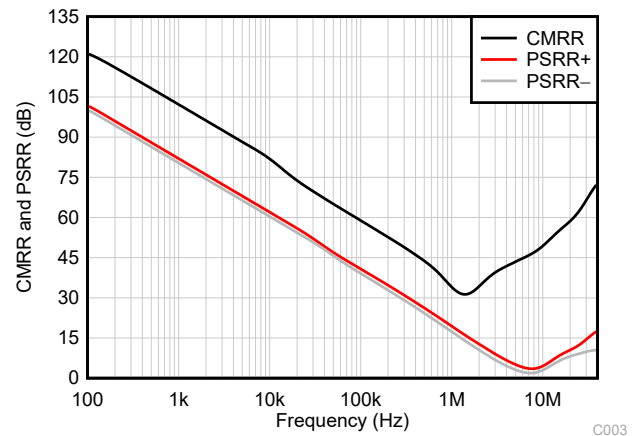
図 5-16. CMRR および PSRR と周波数との関係
