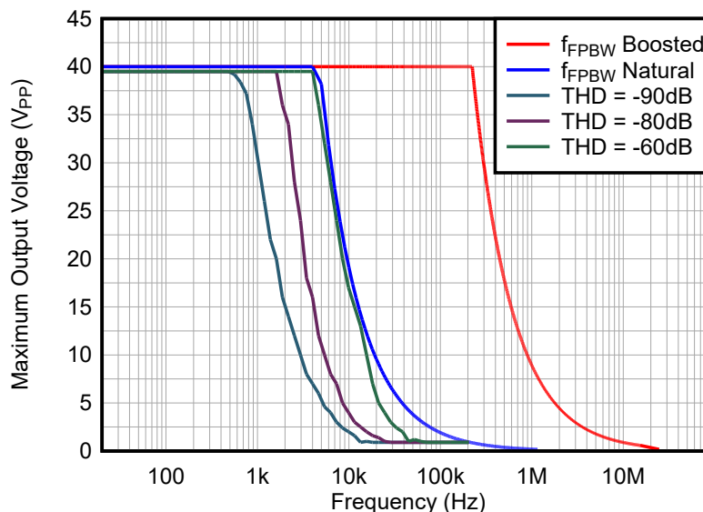
図 7-3. OPAx991-EP の自然環境および昇圧スルーにおける最大出力電圧と周波数との関係
