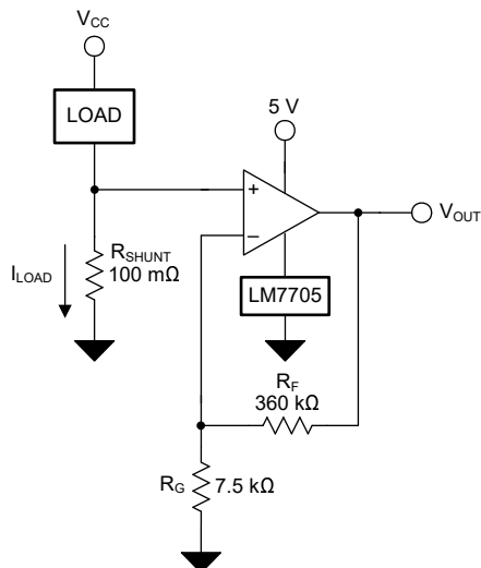
図 7-4. ローサイド電流検出アプリケーションの OPAx991-EP
