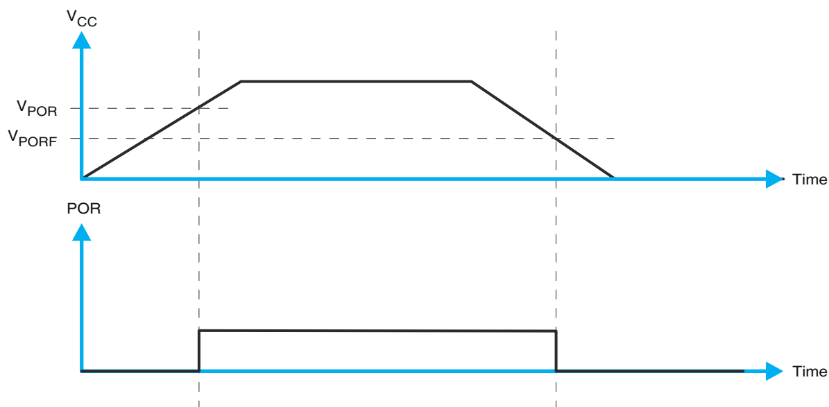
FIG 11-4. V_{POR}
