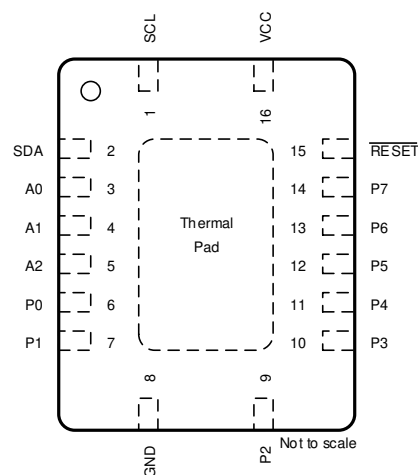
図 4-2. RGY or RGV Package, 16-Pin VQFN or VQFN (Top View)
